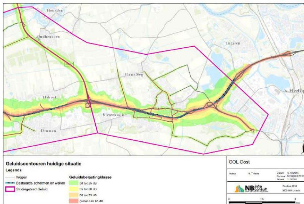
Figuur 6.1 Geluidbelasting huidige situatie. In het achtergrondrapport Geluid is een grotere versie opgenomen.
