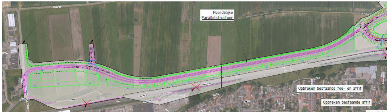
Figuur 4.6 Civiel ontwerp. Noordelijke Parallelstructuur Waalwijk. Paarse lijnen zijn nieuwe wegen. Groene lijnen zijn inpassingsmaatregelen. Het ruimtelijk ontwerp is opgenomen in bijlage 5.
