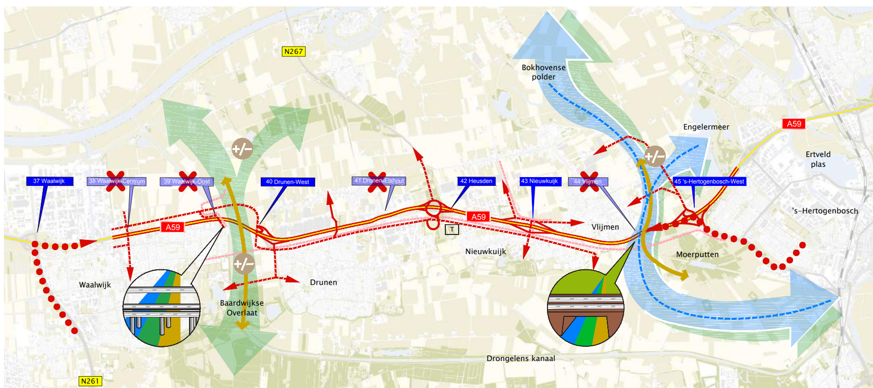
Figuur 1.4 Een schematisch overzicht van het van GOL. In bijlage 1 is een overzicht opgenomen van alle GOL maatregelen.
