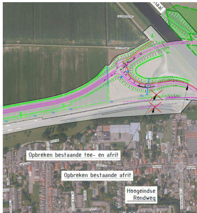
Figuur 4.4 Civiel ontwerp. Aansluiting 39 komt te vervallen. Paarse lijnen zijn nieuwe wegen. Groene lijnen zijn inpassingsmaatregelen. Het ruimtelijk ontwerp is opgenomen in bijlage 5.
