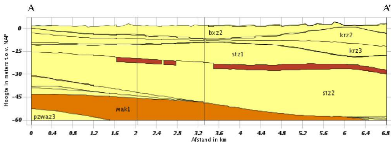
Figuur 3.9: Bodemopbouw langs tracé A- A'.
