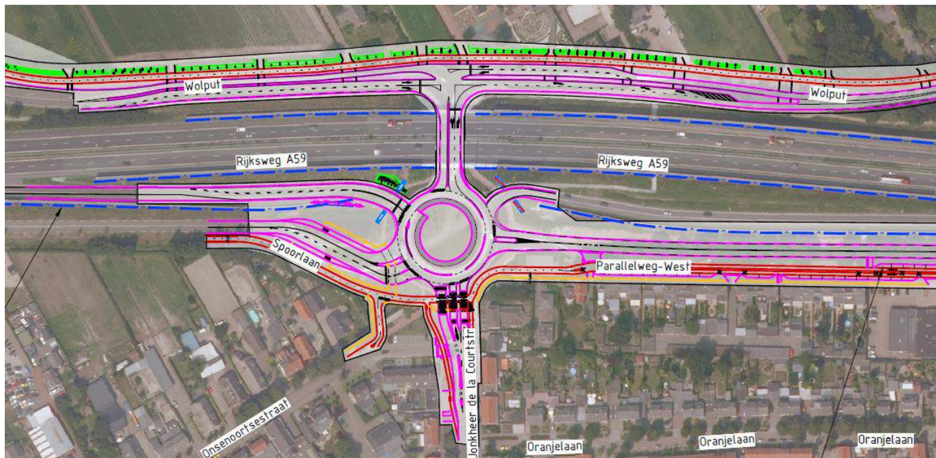
Figuur 4.11 Civiel ontwerp. NRD-alternatief aansluiting 43: de rotonde wordt omgebouwd en de wegen ten noorden en zuiden van de A59 worden aangepast. In fase 2 wordt de parallelweg-west aangelegd. Het ruimtelijk ontwerp is opgenomen in bijlage 5.
