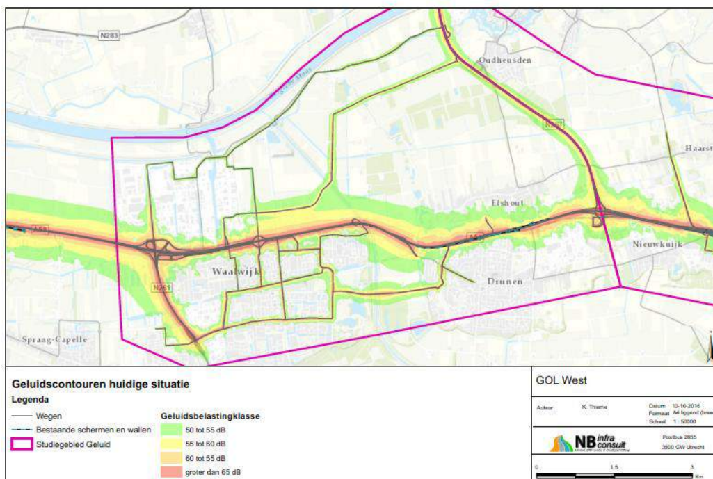
Figuur 6.3 Geluidbelasting huidige situatie. In het achtergrondrapport Geluid is een grotere versie opgenomen.
