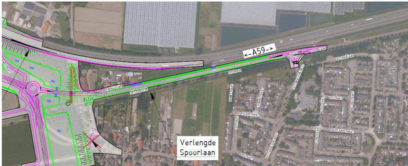
Figuur 4.10 Civiel ontwerp. Doortrekken Spoorlaan. Paarse lijnen zijn nieuwe wegen. Groene lijnen zijn inpassingsmaatregelen. Het ruimtelijk ontwerp is opgenomen in bijlage 5.
