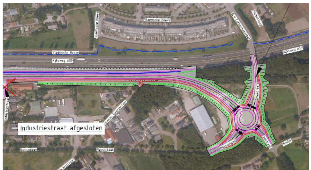
Figuur 4.12 Civiel ontwerp van de variant met verlegde toe- en afrit. De bovenste figuur is de omgeving Nassaulaan. De onderste figuur is de omgeving Vendreef. Het ruimtelijk ontwerp is opgenomen in bijlage 5.
