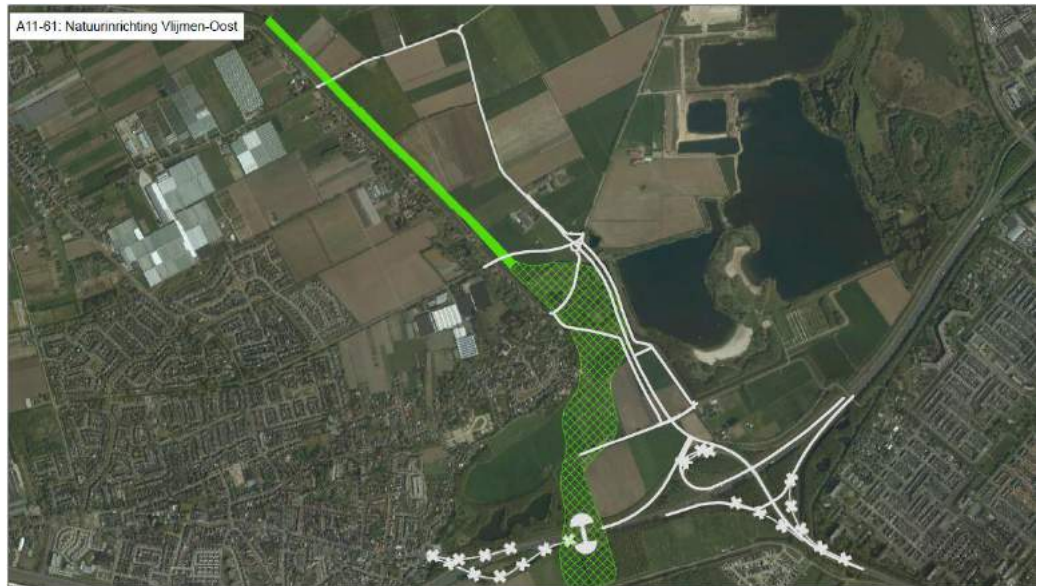
Figuur 4.19 Natuurinrichting Vlijmen Oost: : aanleg Ecologische verbindingszone (EVZ) (groene strook). De witte lijn is een andere GOL-maatregel. Groen geblokte deel is deel van de EVZ dat niet binnen het programma GOL valt.
