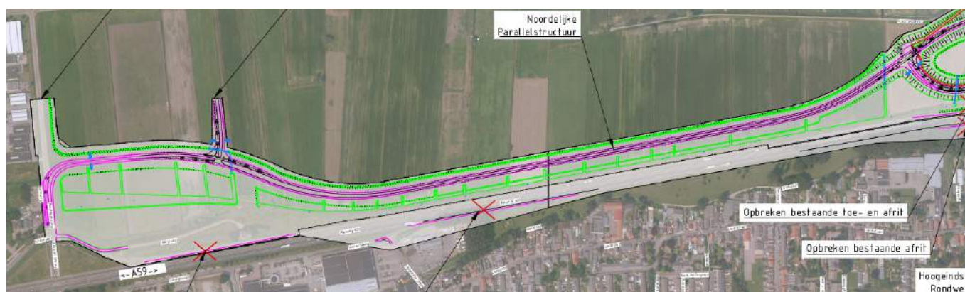
Figuur 4.1 Noordelijke parallelweg bij Waalwijk. Paarse lijnen zijn nieuwe wegen. Groene lijnen zijn inpassingsmaatregelen. De bestaande toe- en afrit 38 en 39 worden afgesloten (weergegeven met een rood kruis in de figuur).
