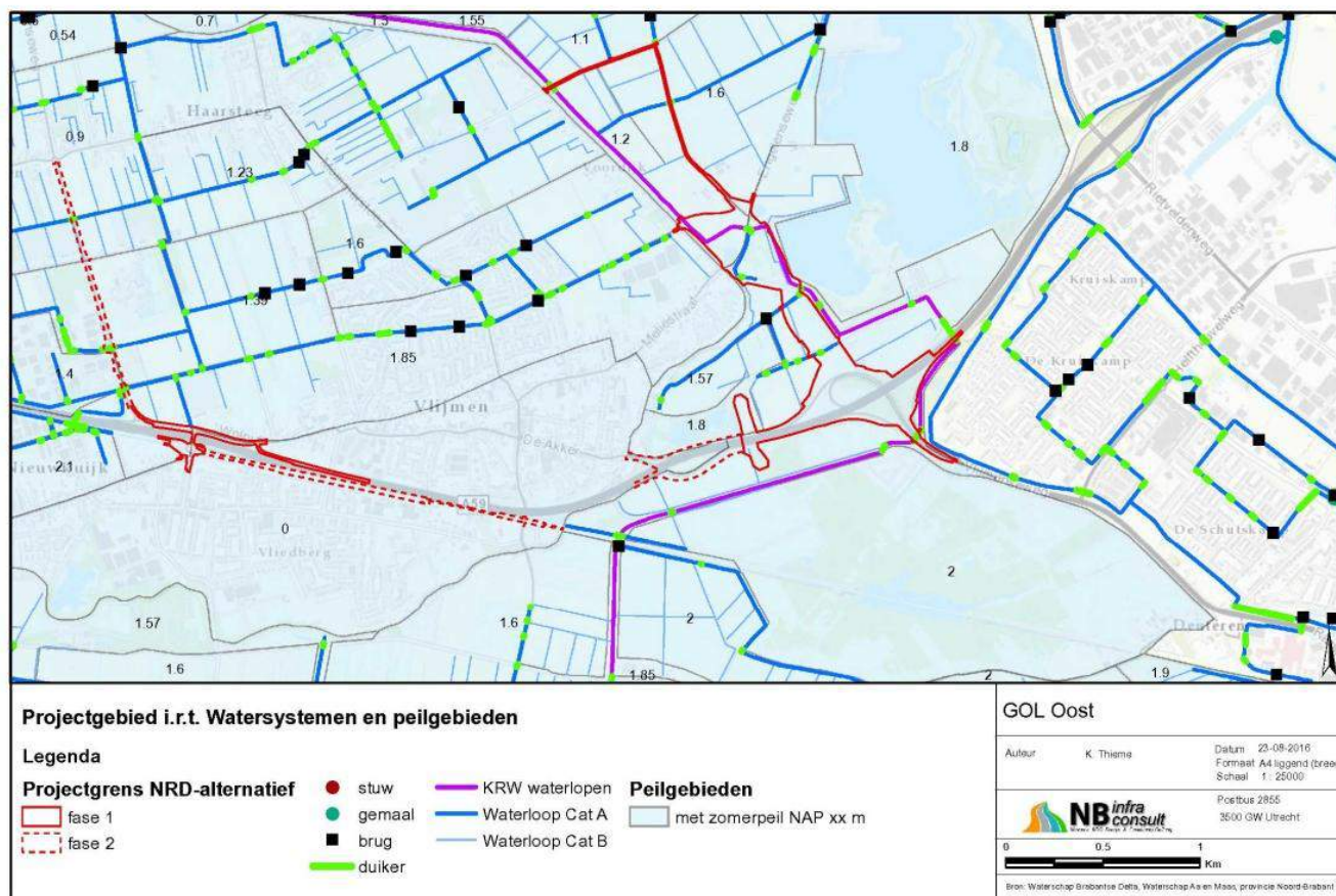
Figuur 3.4: Watersysteem voor GOL Oost.
