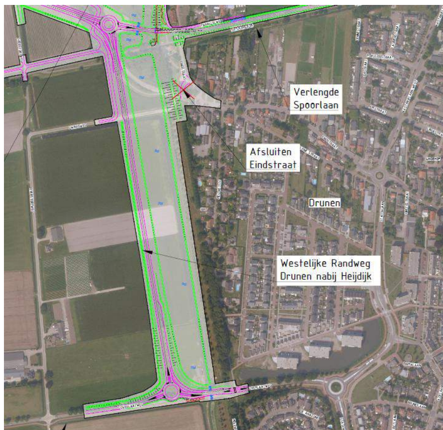
Figuur 4.7A Civiel ontwerp. Westelijke Randweg Drunen nabij Heijdijk. Paarse lijnen zijn nieuwe wegen. Groene lijnen zijn inpassingsmaatregelen. Het ruimtelijk ontwerp is opgenomen in onderstaande figuur en in bijlage 5.
