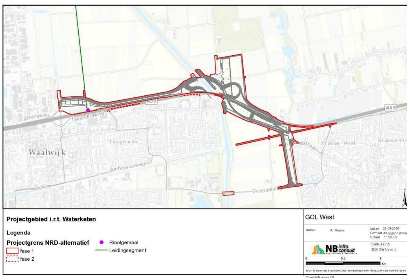
Figuur 5.2: Waterketen objecten.
