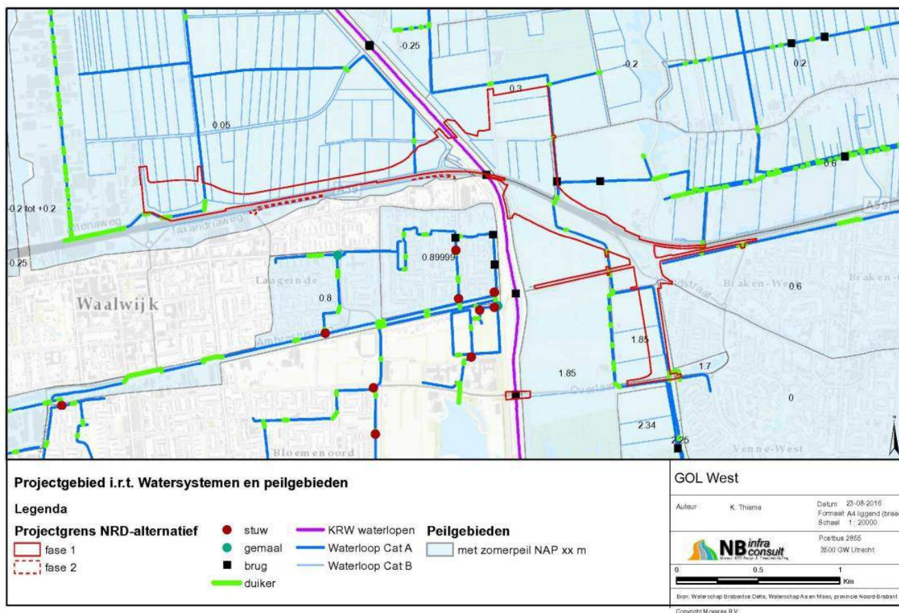
Figuur 3.8: Watersysteem voor GOL West.
