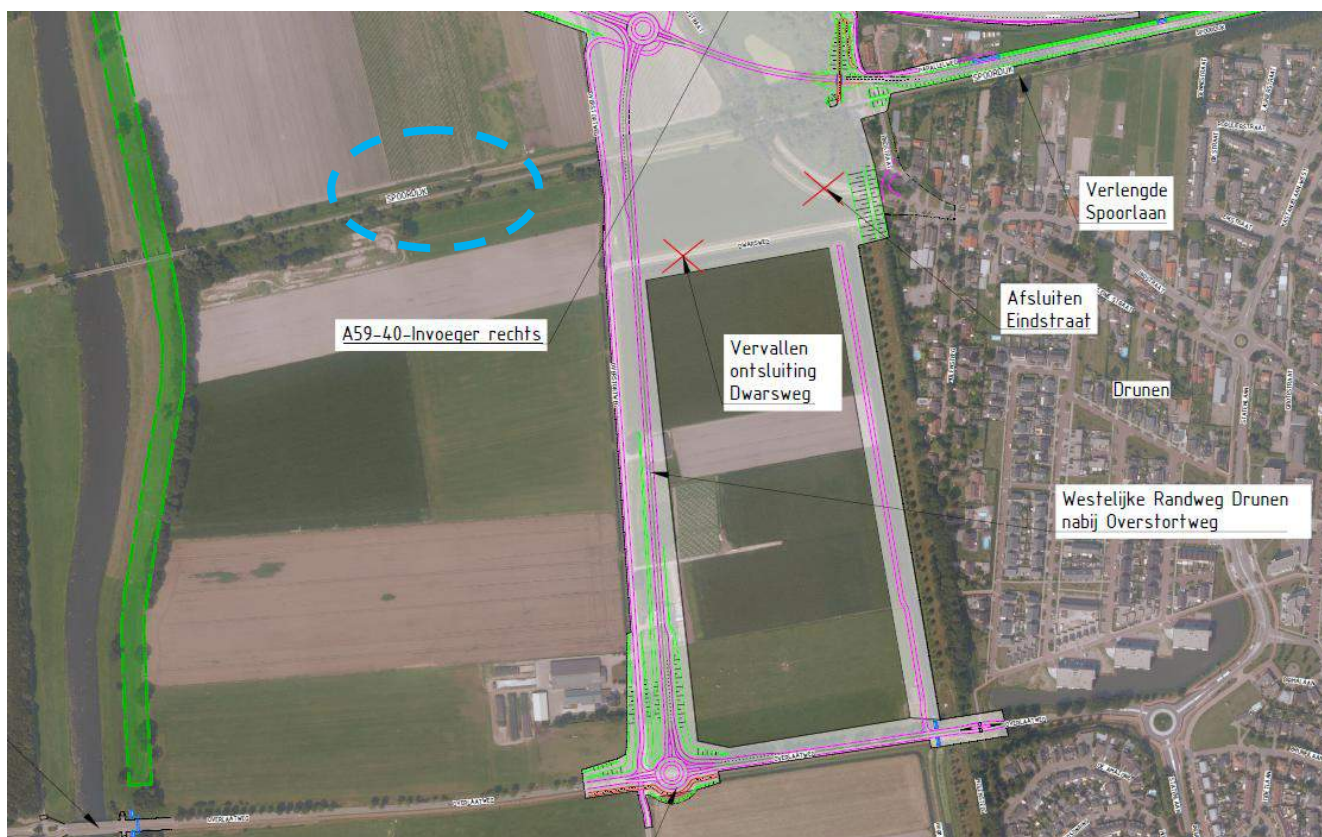
Figuur 4.8 Civil ontwerp. Variant westelijke randweg Drunen nabij Overstortweg. Paarse lijnen zijn nieuwe wegen. Groene lijnen zijn inpassingsmaatregelen. Het open te maken deel van de spoordijk is indicatief weergegeven met een blauwe gestippelde cirkel. Het ruimtelijk ontwerp is opgenomen in bijlage 5.
