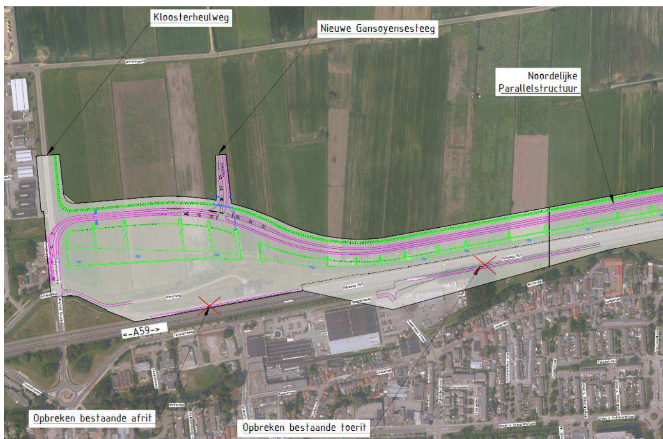
Figuur 4.3 Civiel ontwerp. Aansluiting 38 komt te vervallen. Paarse lijnen zijn nieuwe wegen. Groene lijnen zijn inpassingsmaatregelen. Het ruimtelijk ontwerp is opgenomen in bijlage 5.
