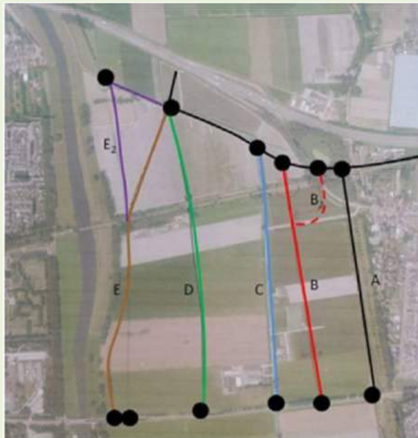
Onderzochte tracés in de Baardwijkse Overlaat
