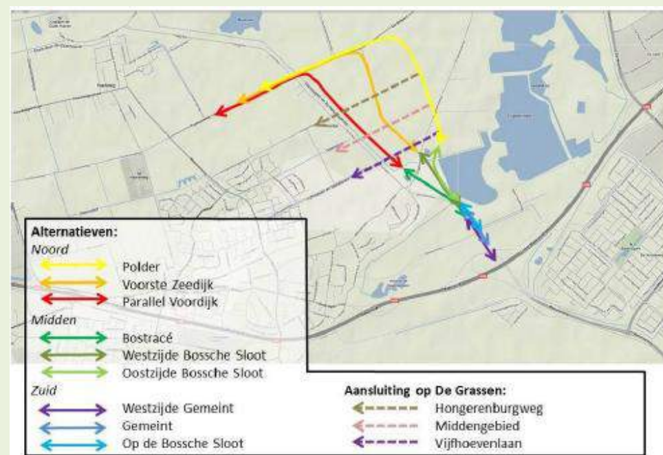
Onderzochte tracés voor de Randweg Vlijmen
