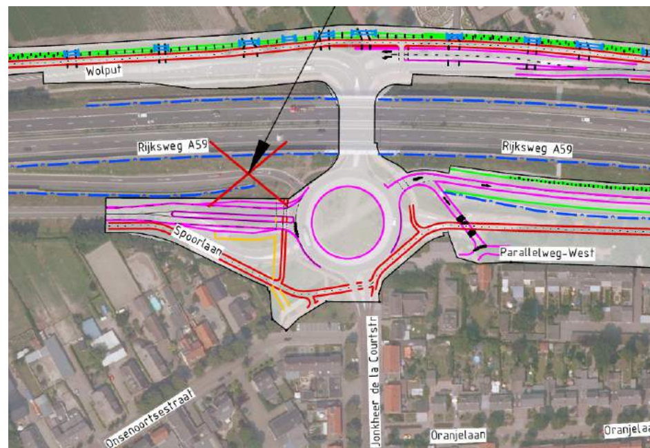
Figuur 3.3 Het principe van de turborotonde in het NRD-alternatief inclusief aanpassingen aan de omliggende wegen. Een turborotonde is een rotonde met meer dan één rijstrook op de rotonde. De vormgeving is dusdanig dat voertuigen als vanzelf van de binnenste naar de buitenste rijstrook worden geleid om de rotonde te verlaten.
