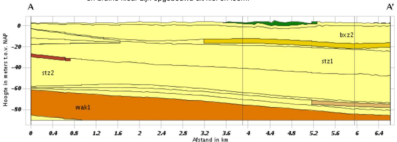
Figuur 3.5: Bodemopbouw langs tracé A- A'.
