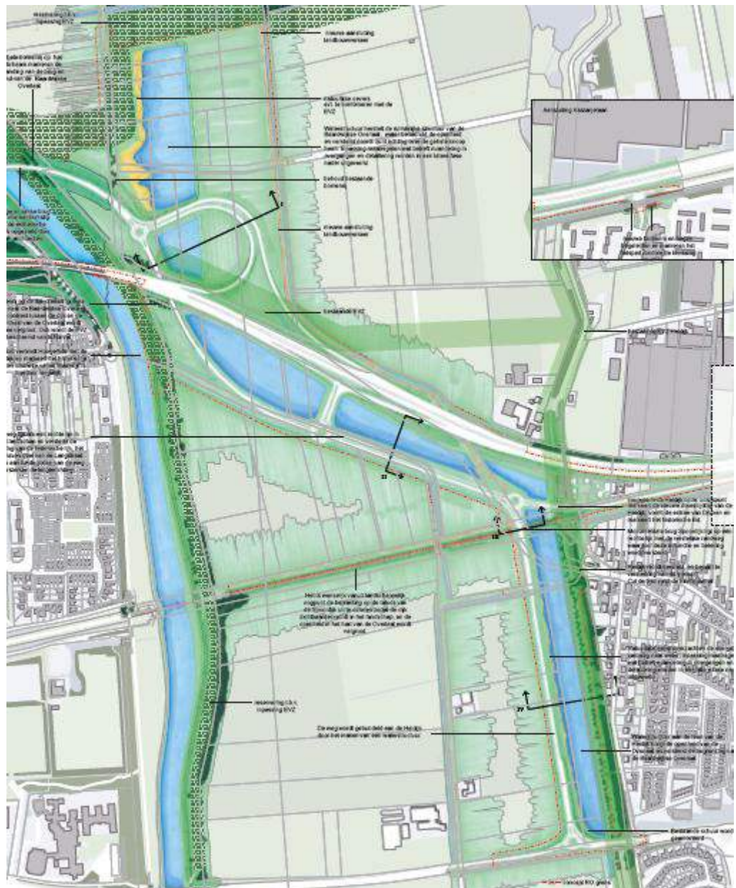
Figuur 21B. Ruimtelijk Ontwerp. Westelijke Randweg Drunen nabij Heidijk met de ligging van de waterslinger. Een grotere versie van deze figuur is opgenomen in bijlage 5.
