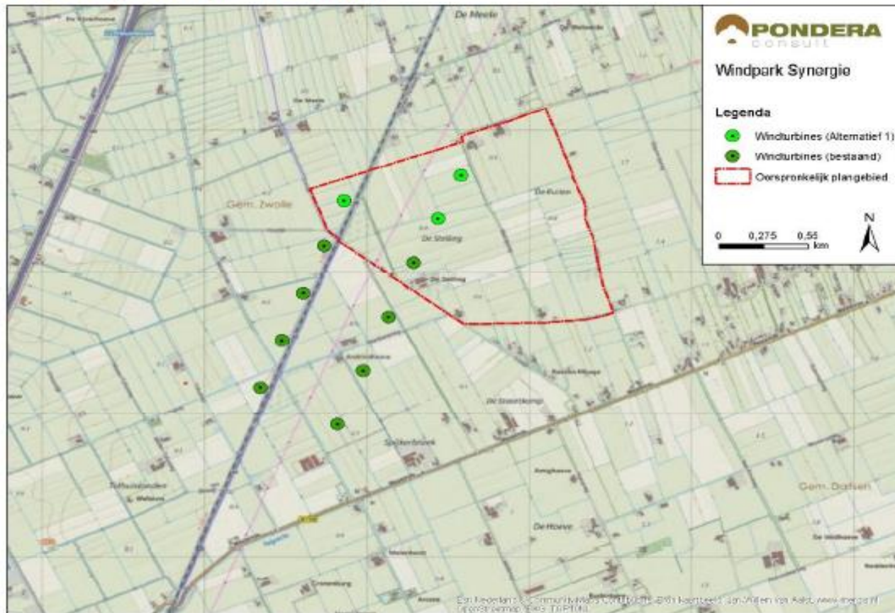
Figuur S.2 Illustratie alternatief 1: windpark met vergelijkbare windturbines als in bestaande windparken (uitbreiding bestaande lijnen)
