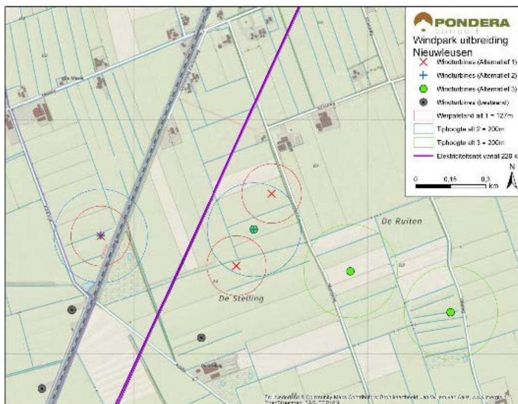
Figuur 11.4 Hoogspanningsverbinding in relatie tot toetsafstanden
