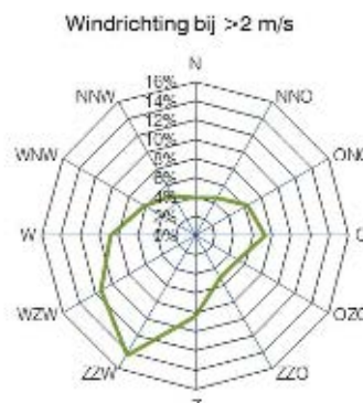
Figuur 3.2 Distributie windrichtingen
