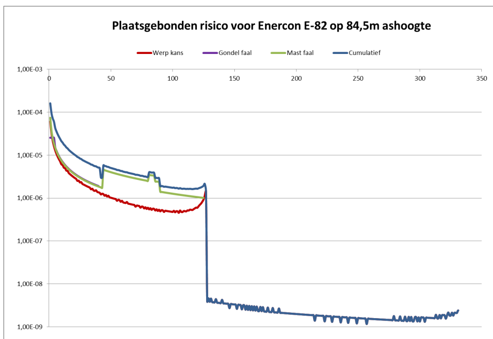
Figuur 1.4 Plaatsgebonden Risico (PR) voor Enercon E-82 op 84,5 meter ashoogte
