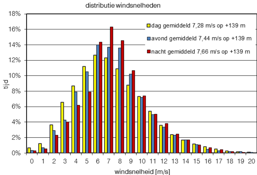
Figuur 2.2 Distributie van de voorkomende windsnelheden op ashoogte +139m
