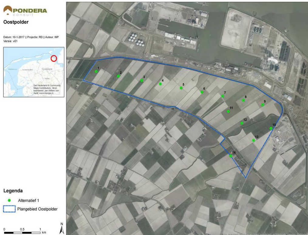
Abbildung 1.4 Aufstellung Alternative 1
