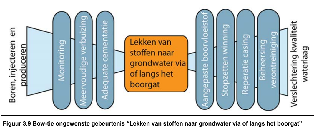
Figuur 3.9 Bow-tie ongewenste gebeurtenis “Lekken van stoffen naar grondwater via of langs het boorgat”
