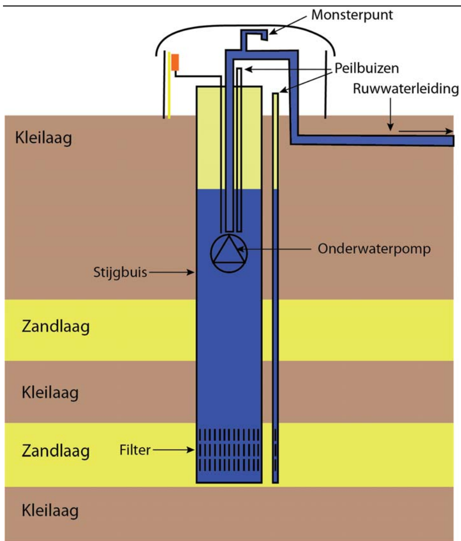
Figuur 3.4 Schematische weergave van een grondwaterwinput
