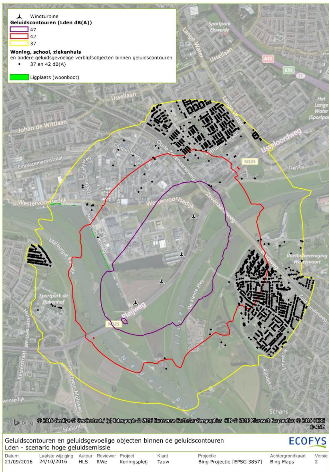
Figuur I.1. Ligging windpark en geluidcontouren 'normaal' geluid.
