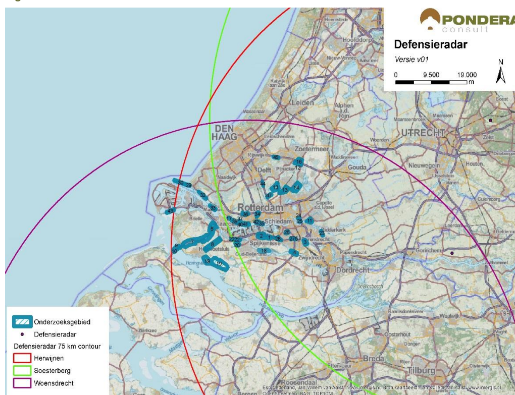
Figuur 3.4 Defensieradar
