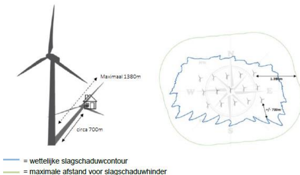
Figuur 3.1 Van norm naar afstanden slagschaduw
