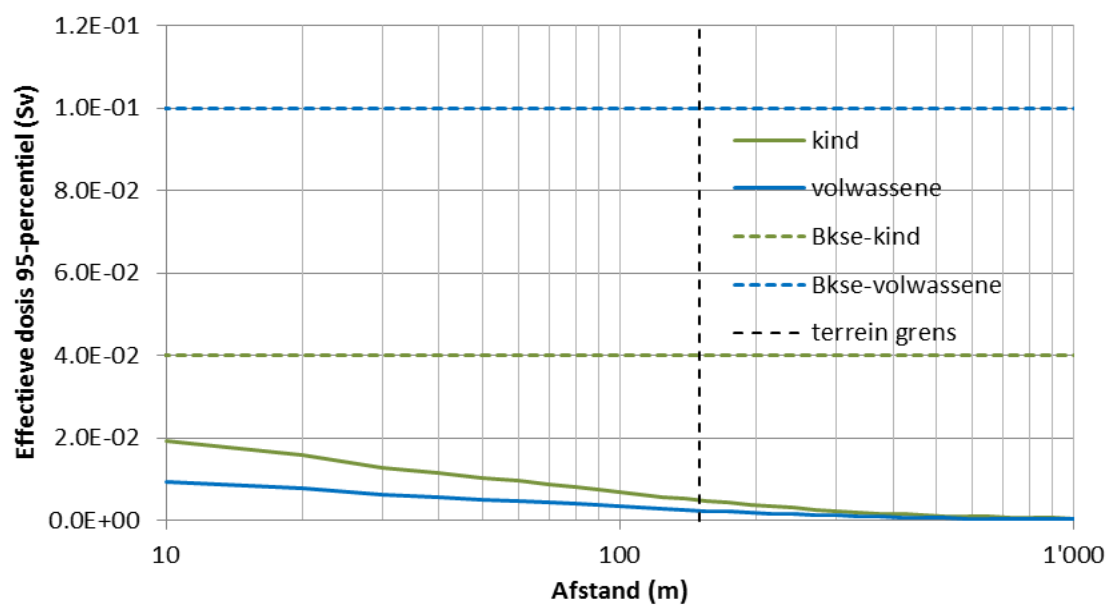
Figuur G.3 Maximale dosis als functie van de afstand bij het ontwerpgeval 'Systeemlek van een tank met hoog-radioactief vloeibaar afval'
