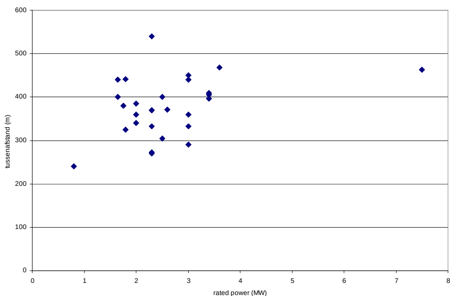
Figuur b.1: Relatie tussen vermogen van turbines (rated power, in MW) en tussenafstanden bij bestaande en concreet geplande windparken in (overwegend) Flevoland en Noord-Holland
