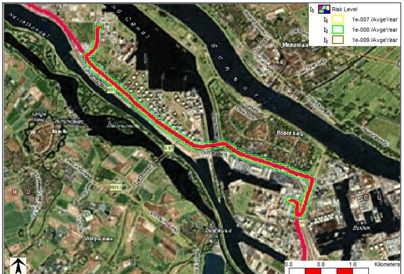
Figuur 23: Traject 4, plaatsgebonden risico oxogasleiding
