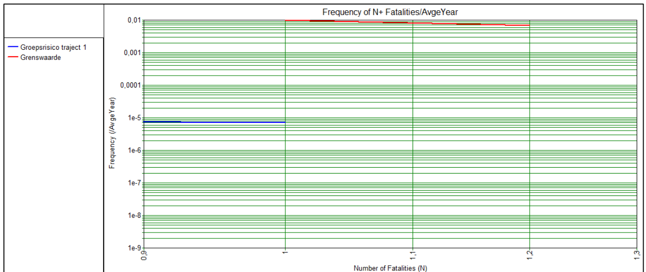
Figuur 4: Traject 1, groepsrisico, kilometer met hoogste groepsrisico
