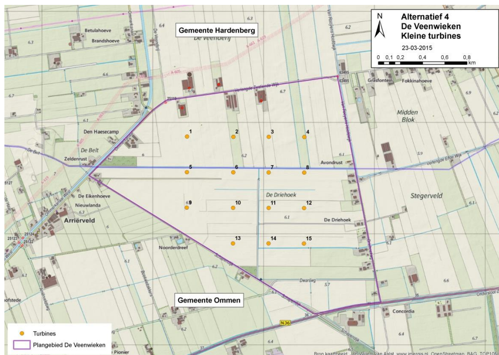
Figuur S7 Alternatief 4: kleinere windturbines
