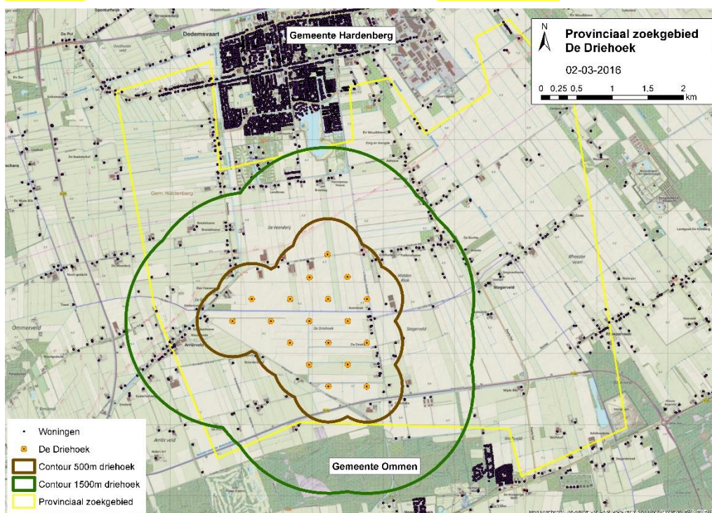
Figuur 3.13 Contouren van 500 meter en 1500 meter rond de opstelling locatie de Driehoek
