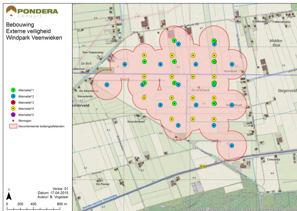
Figuur 11.2 Veiligheidsafstand bij bebouwing
