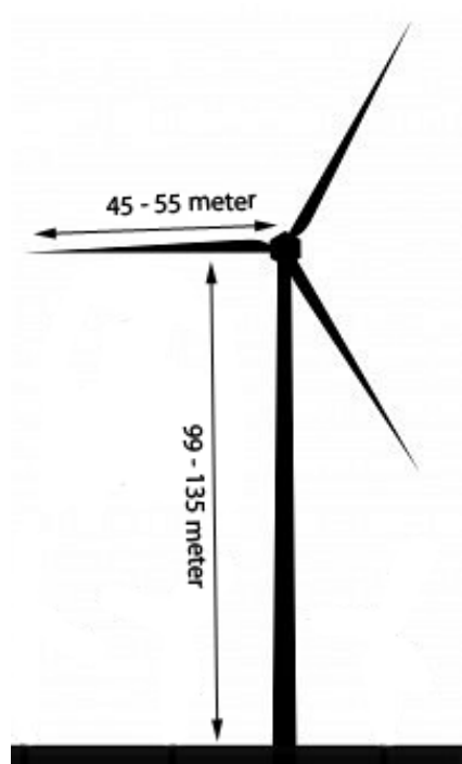
Figuur 4.2 Illustratie afmetingen
