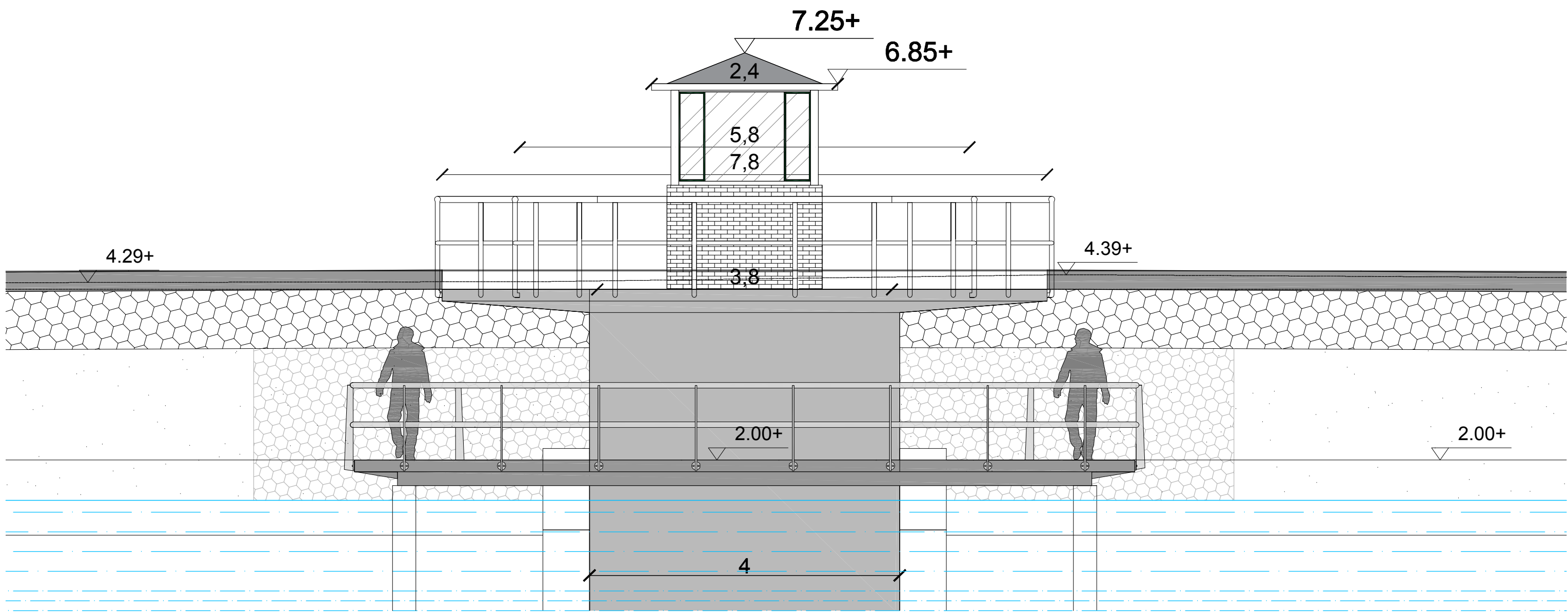
Voorraanzicht van de stalen vlinder rond het Hanepraagemaal, schaal 1 : 50
