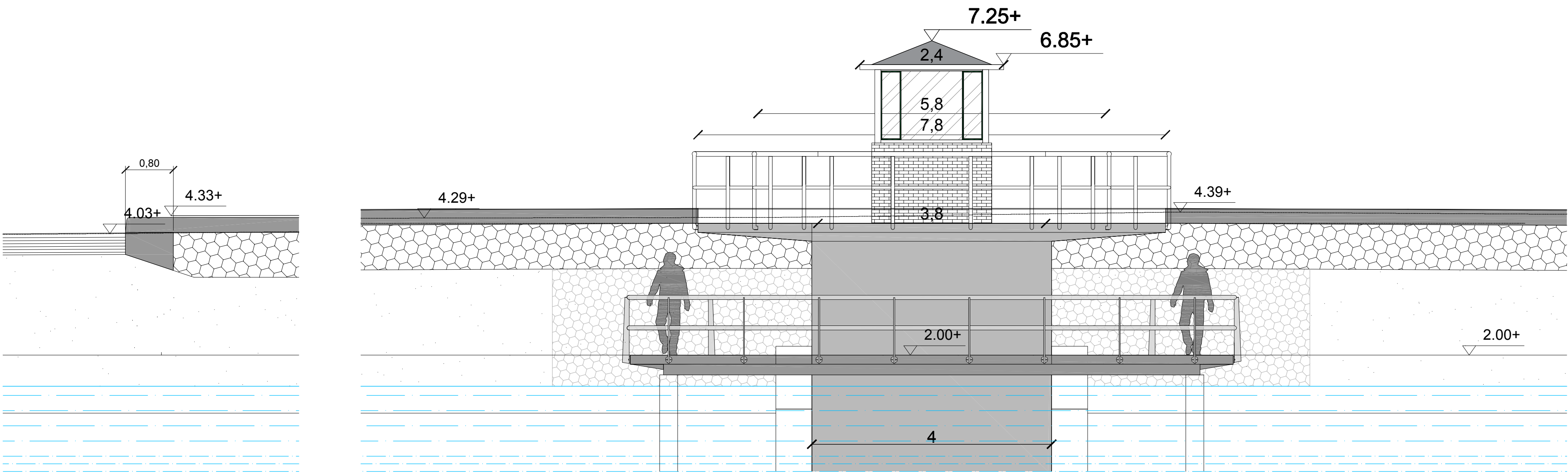
Betonnen eindblok bij aansluiting op de bestaande gemetselde muur, schaal 1 : 50
