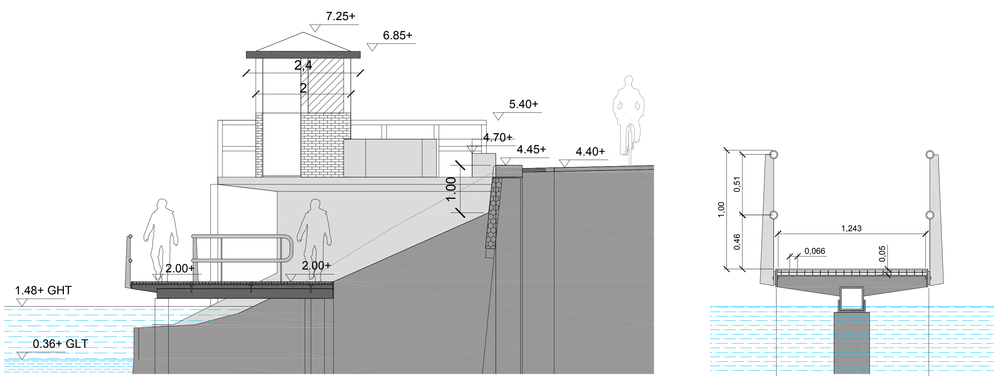
Doorsnede aanzicht van de stalen vlinder rond het Hanepraagemaal, schaal 1 : 50
