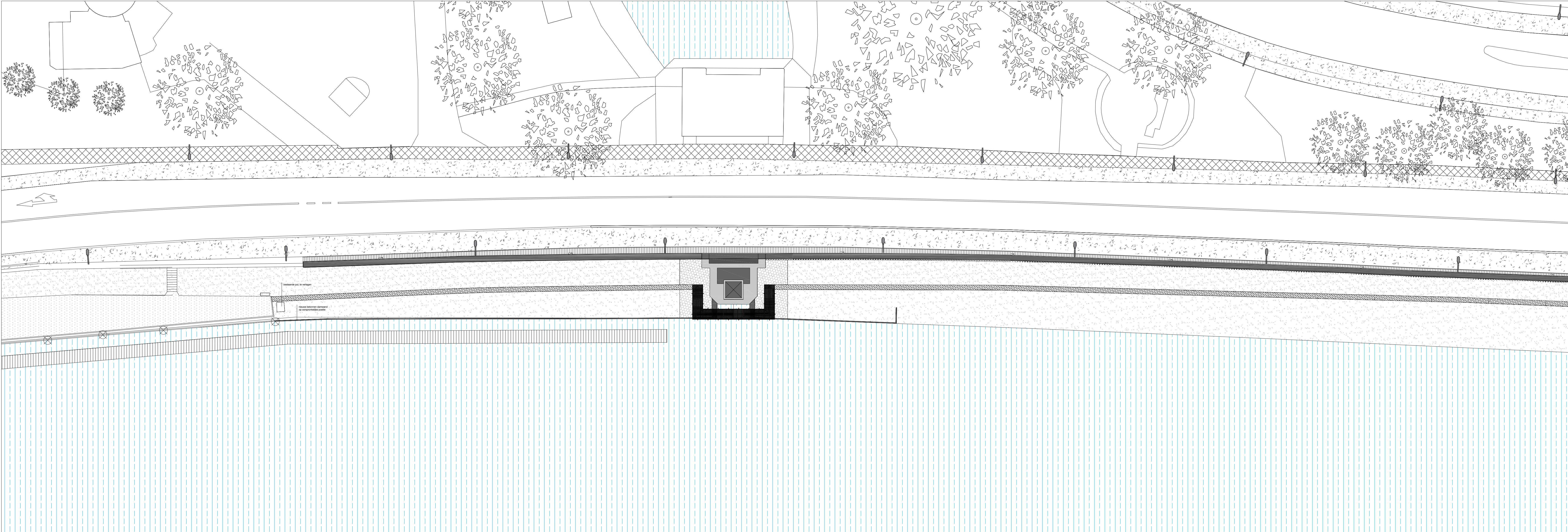
Bovenaanzicht van de stalen vlinder rond het Hanepraagemaal, schaal 1:50
