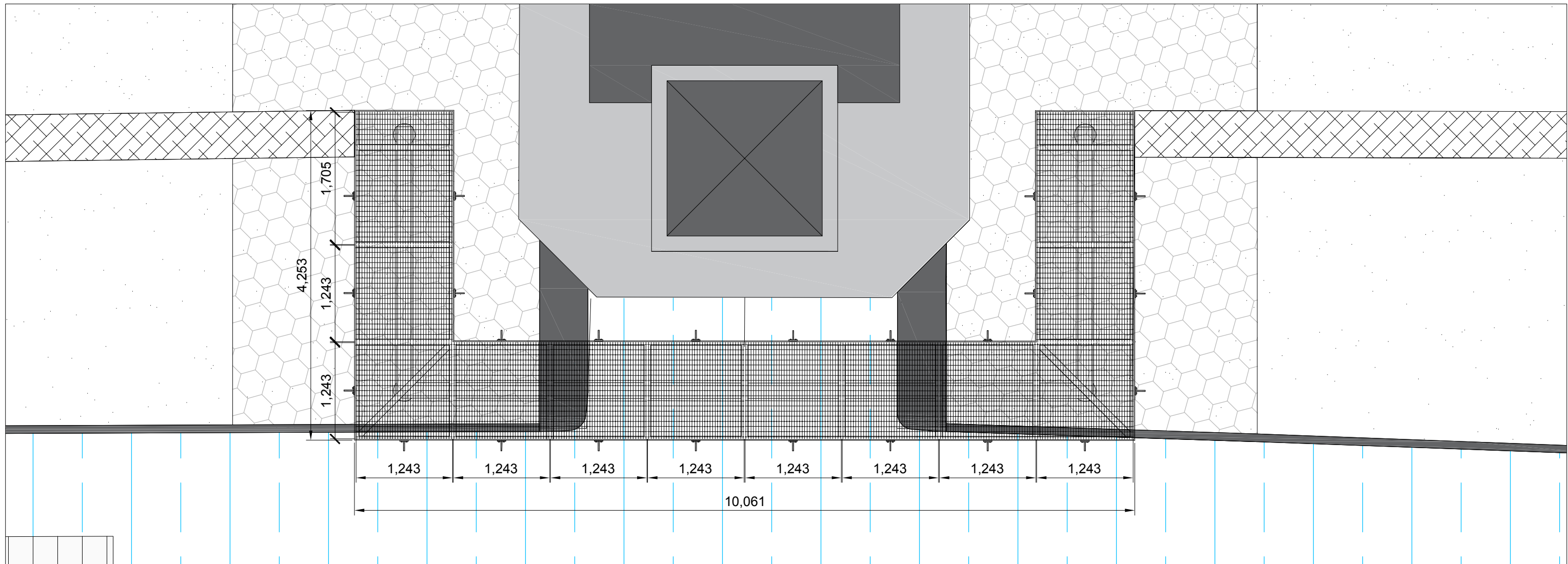
Bovenaanzicht van de stalen vlinder rond het Hanepraagemaal, schaal 1:50
