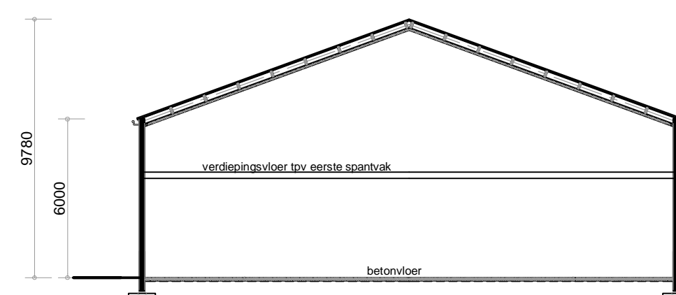
- Doorsnede C - C gebouw 2 -
