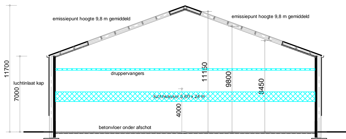
- Doorsnede A - A gebouw 3 en 4 -
