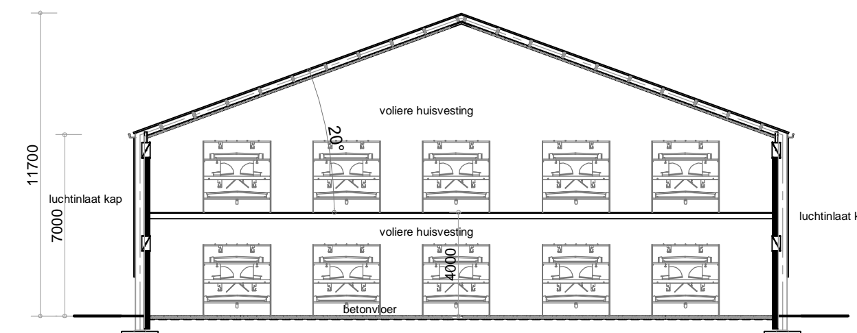
- Doorsnede B - B gebouw 3 en 4 -
