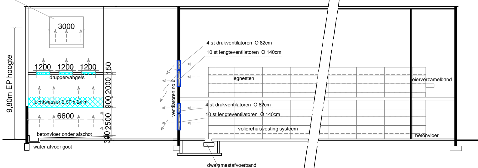
- Langsdoorsnede gebouw 3 en 4 -
