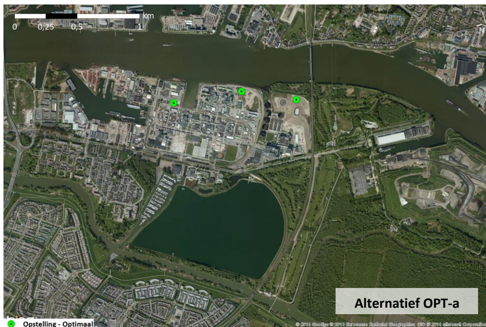
Figuur 16: Alternatief OPT-a De fysieke ruimte op het bedrijventerrein maakt een rechte lijn van drie windturbines parallel aan de rivier 'Beneden Merwede' niet mogelijk.
