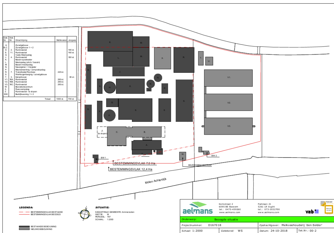
Figuur 1: Voorgenomen bedrijfsvernieuwing; de lichtgrijze delen zijn nieuw ten opzichte van de huidige situatie (bron: MER)
