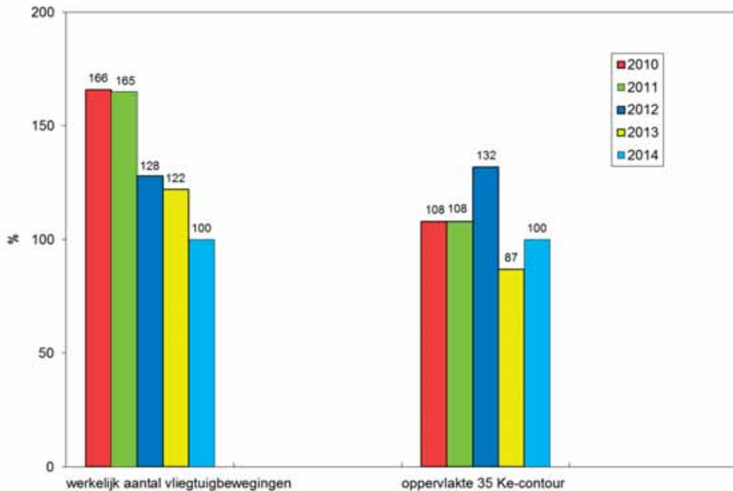
Figuur 5: Percentage vliegtuigbewegingen (exclusief nachtstraffactor) en oppervlakte van de 35 Ke-contour, beide ten opzichte van het jaar 2014 (=100%), Vliegbasis Woensdrecht
