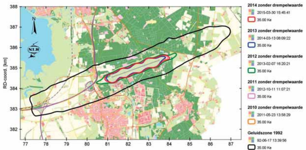
Figuur 4: 35 Ke-geluidbelastingscontouren voor de jaarberekeningen zonder drempelwaarde voor de jaren 2010 tot en met 2014
