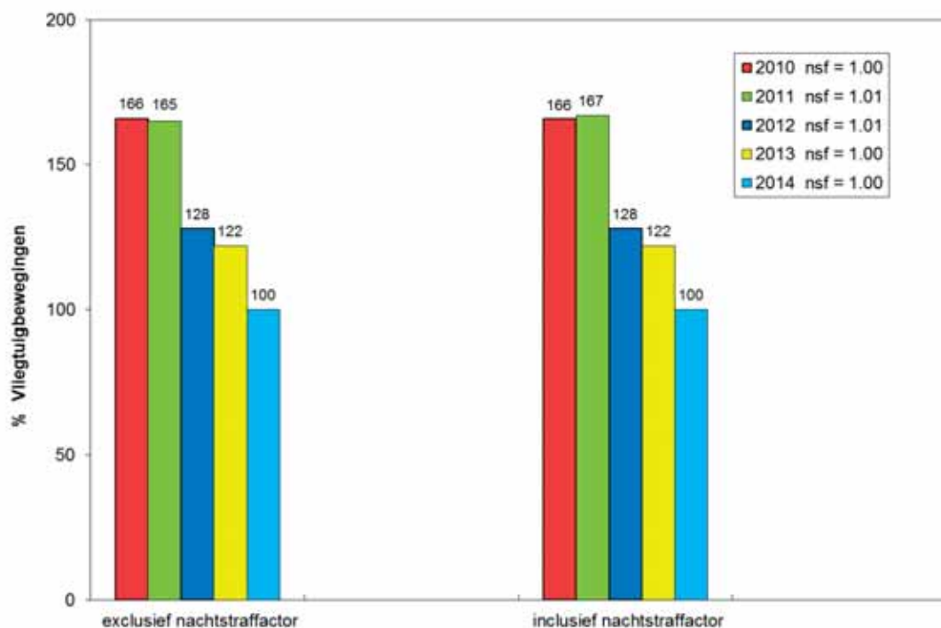
Figuur 1: Percentage vliegtuigbewegingen ten opzichte van het jaar 2014 (exclusief nachtraffactor = 100%), Vliegbasis Woensdrecht
