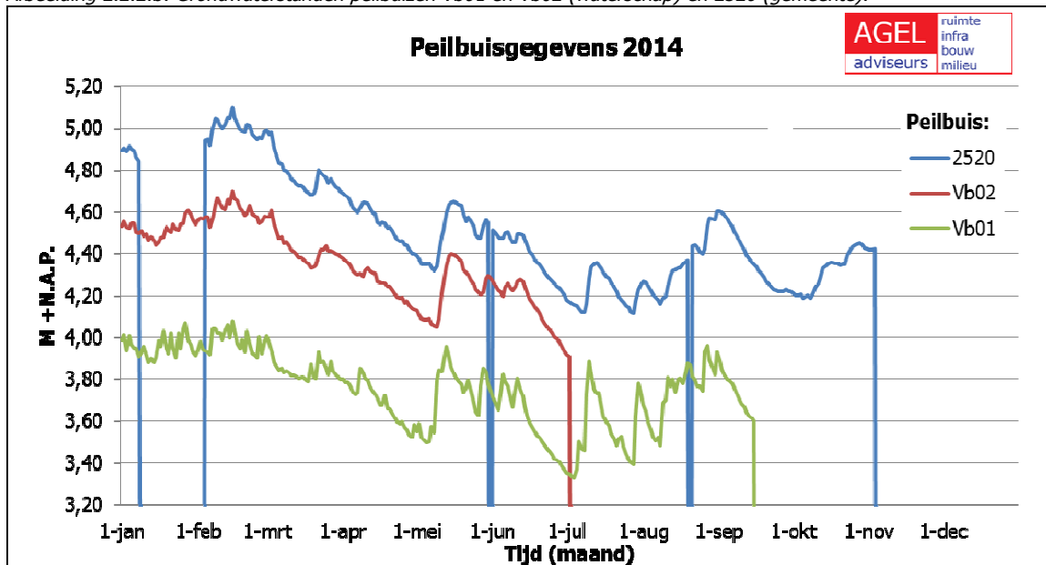
Afbeelding 2.2.2.b: Grondwaterstanden peilbuizen Vb01 en Vb02 (waterschap) en 2520 (gemeente).
