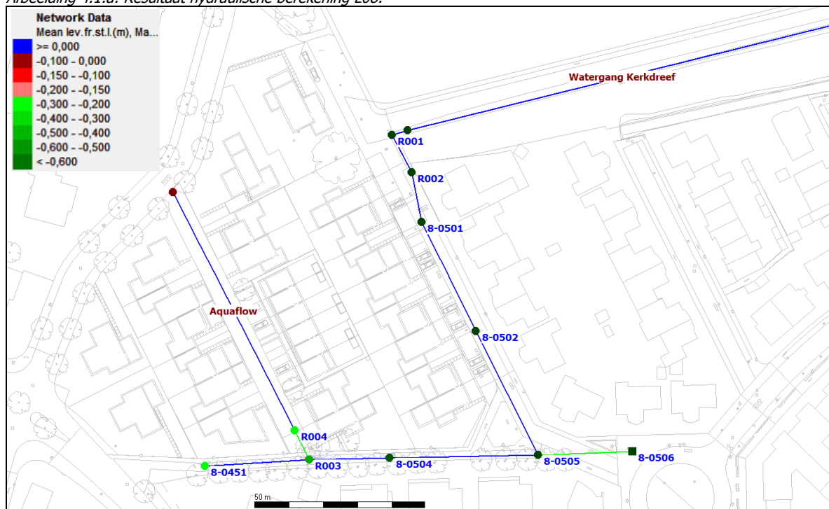
Afbeelding 4.1.a: Resultaat hydraulische berekening L08.
