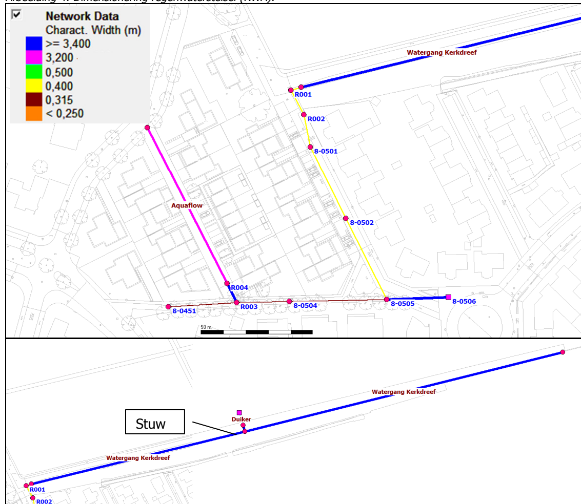
Afbeelding 4: Dimensionering regenwaterstelsel (RWA).
