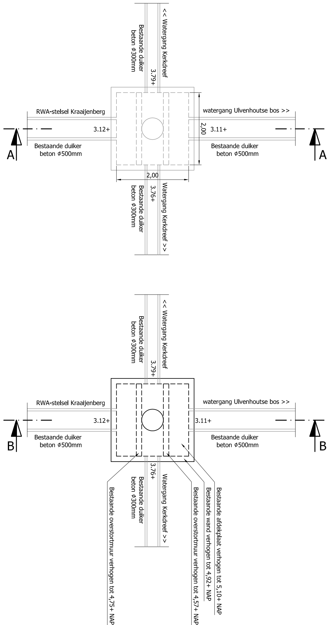
DETAIL 5 (PUT 8-0710 bestaande overstortput) BOVENAANZICHT 1:50
