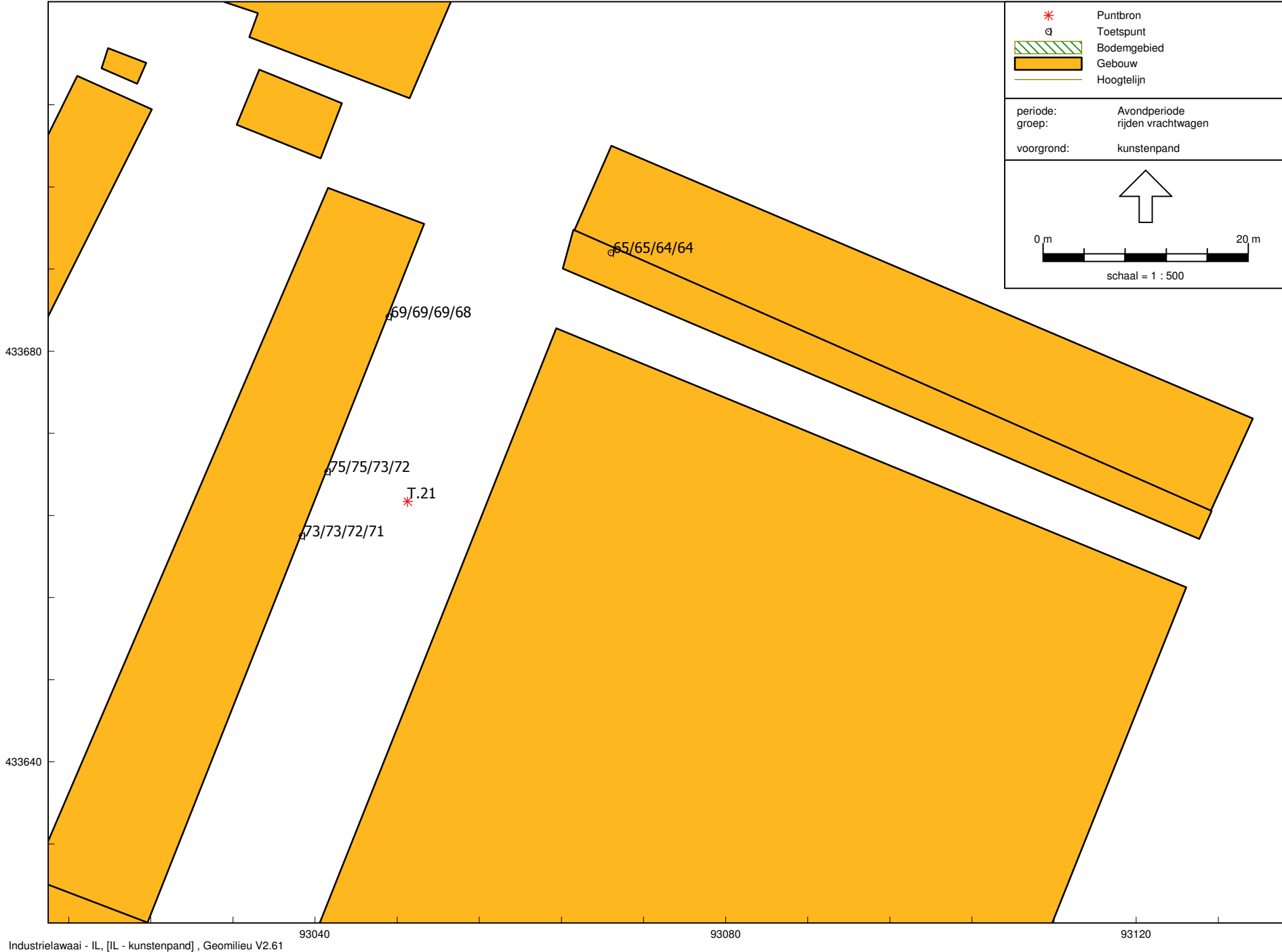
Piekgeluid vanwege laden en lossen bij het kunstenvand in de avondperiode
