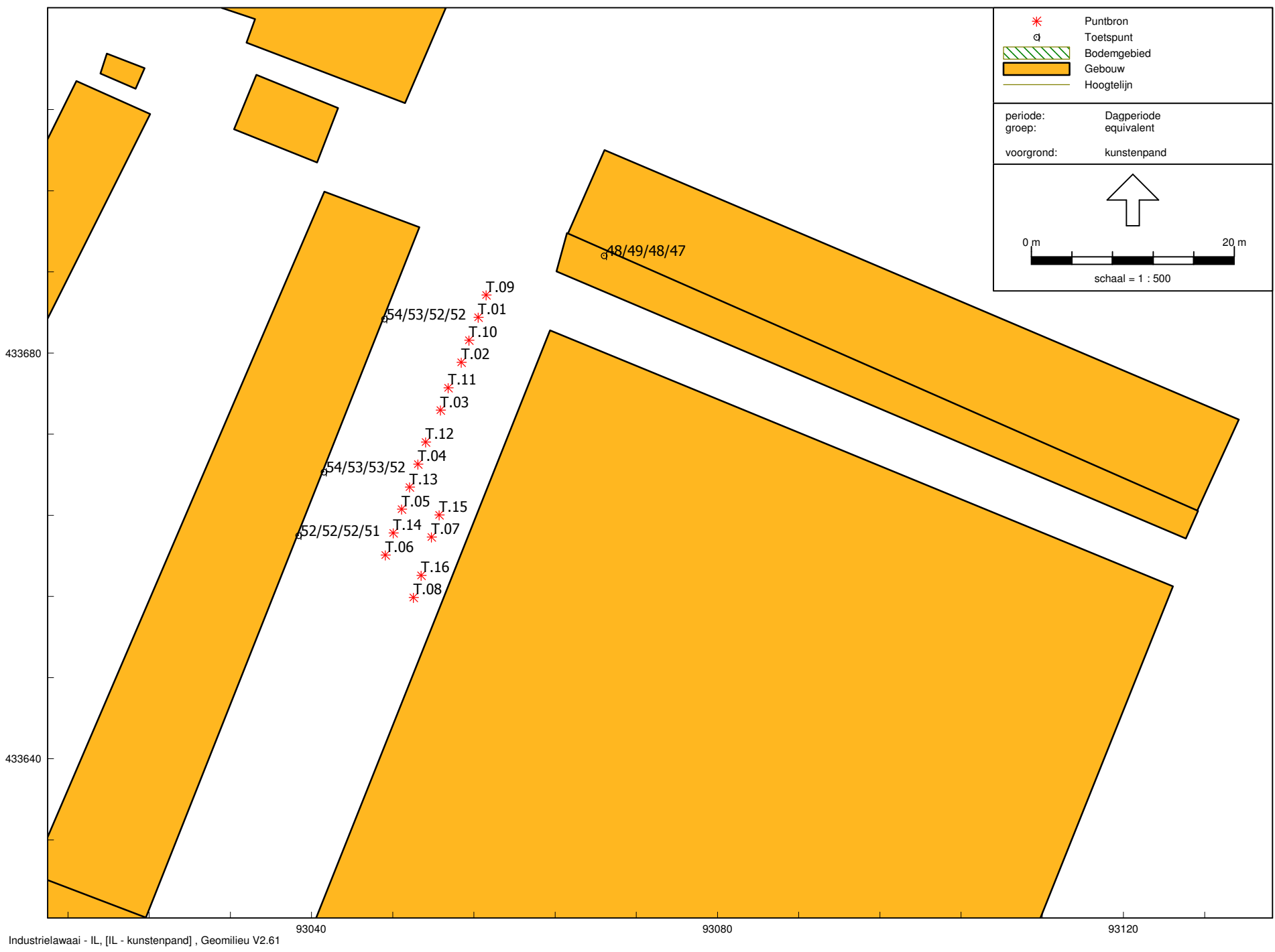
Geluidsbelasting LAR,LT in de dagperiode vanwegeaanrijden naar expeditie van het kunstenvand
