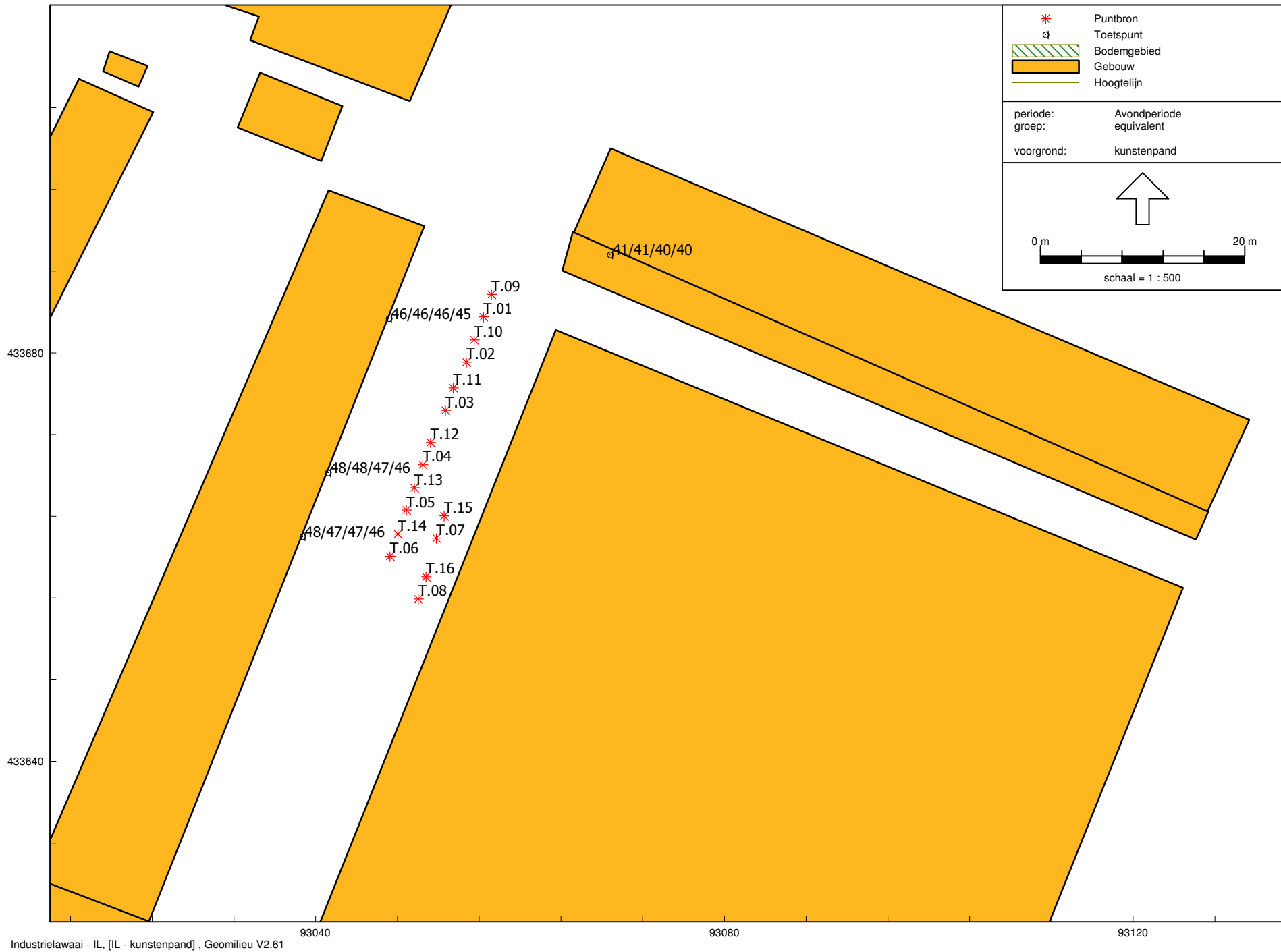
Geluidsbelasting LAR,LT in de avondperiode vanwege wegrijden vanuit de expeditie van het kunstenpand
