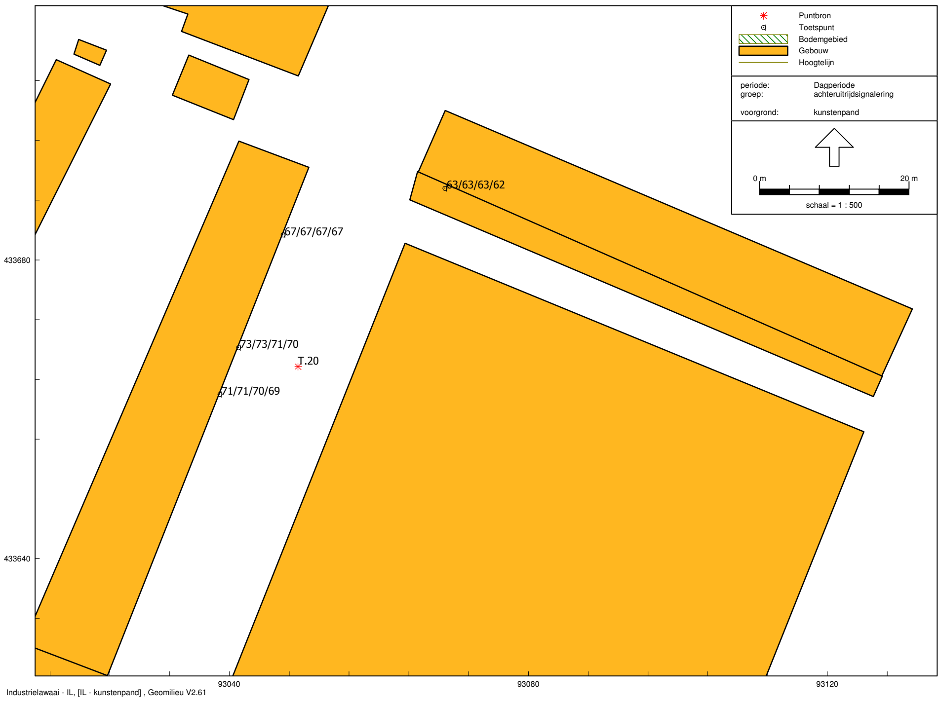
Piekgeluid vanwege laden en lossen bij het kunstenspand in de dagperiode
