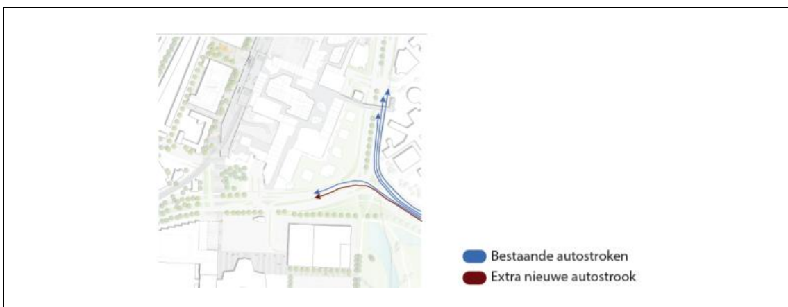
Afbeelding 3.22. Extra linksafstrook Vaanweg
