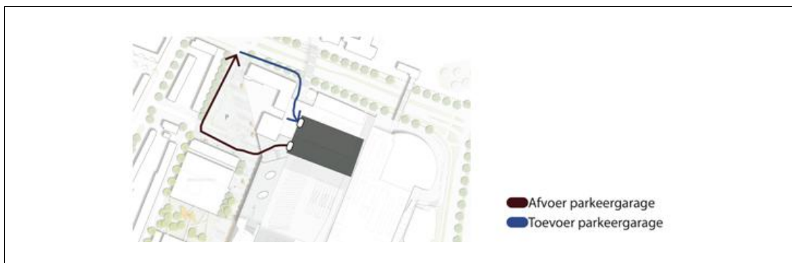
Afbeelding 3.20. Uitbreiding parkeergarage Zuidplein aansluiten op de Pleinweg
