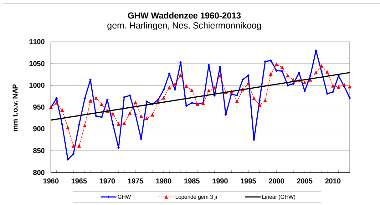
Figuur 3.10 Jaargemiddelde hoogwater van 1960-2013. (Op basis van RWS-data voor Harlingen, Nes en Schiermonnikoog.)
