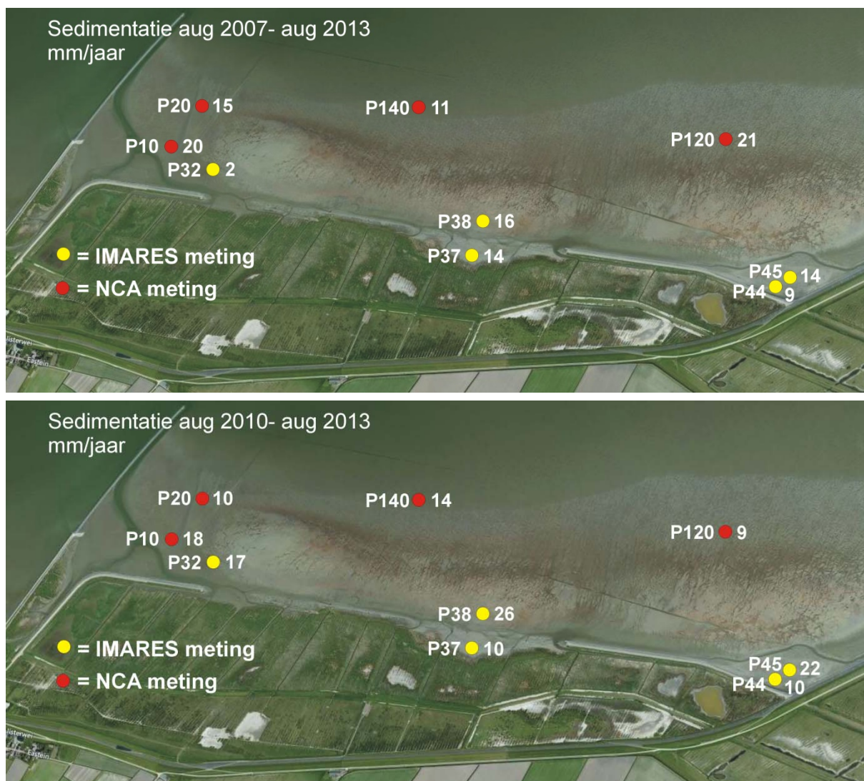
Figuur 3.4. Vergelijking van de opslibningsmetingen van NCA (rode punten) en IMARES (gele punten) op de grens van kwelder en wad bij de Peazemerlannen. Boven over periode aug 2007-aug 2013. Onder over periode aug 2010-aug 2013. De P met nummer betreft het meetpunt en het getal achter de stip de opslibbing in mm/j. Figuur gemaakt door Johan Krol (NCA).
