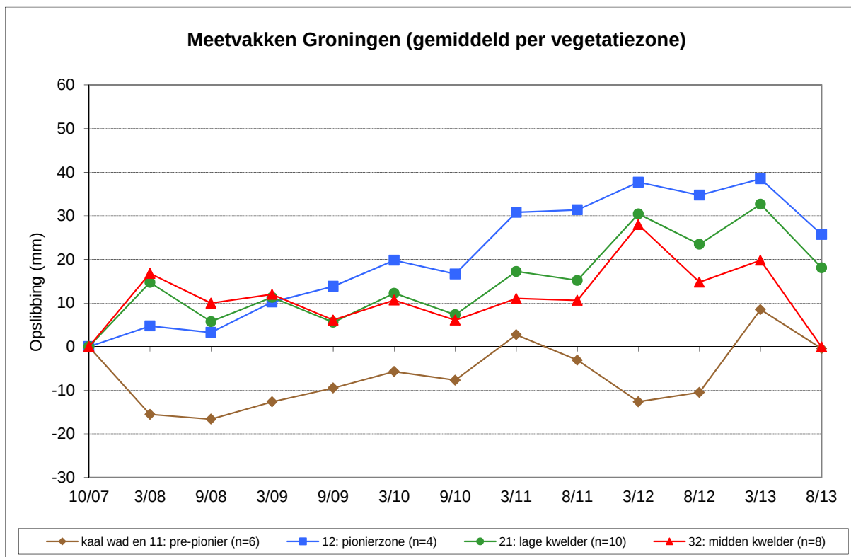
Figuur 3.5 Maaiveldhoogteontwikkeling (mm+NAP) bij de meetpunten in de onderscheiden kwelderzones (met SAL797 code) in het referentiegebied west-Groningen vanaf 2007-augustus 2013.
