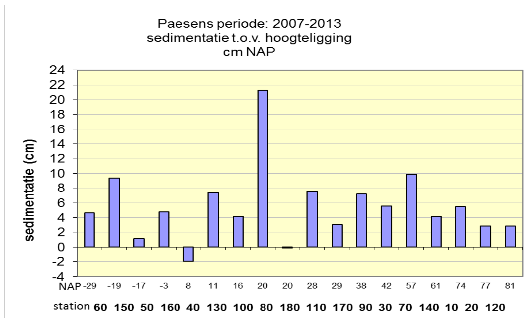
Figuur 29. Sedimentatie P10 – P180 in relatie tot de hoogteligging.
