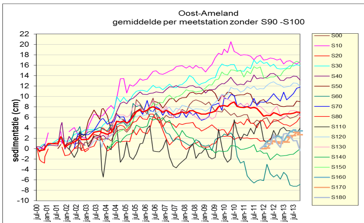
Figuur 20. Gemiddelde meetlijnen van de meetstations S00 tm S80 en S110 tm S180 in het onderzoeksgebied Oost-Ameland. De stations S160 tm S180 starten in 2012. Station S90 en S100 zijn weggelaten. S100 is in 2009 verloren gegaan en S90 is een geulwandstation en niet representatief voor plaatsedimentatie..
