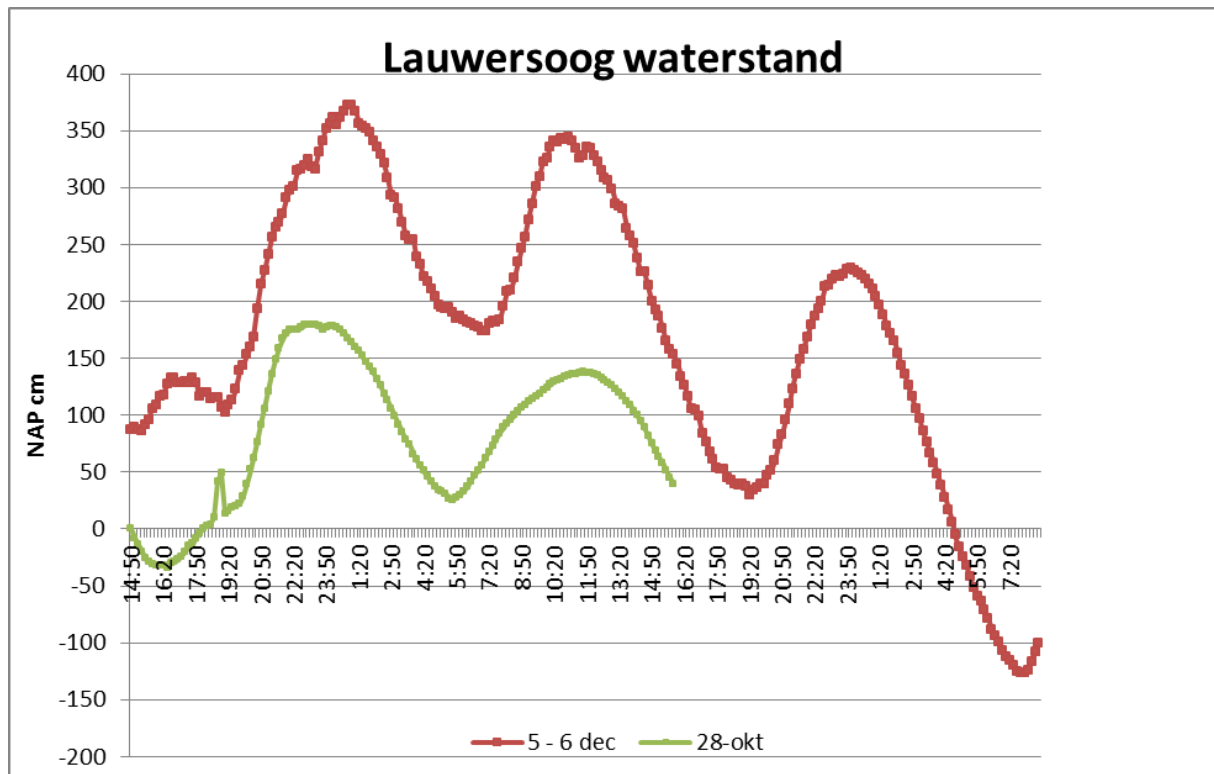
Figuur 34. Het verloop van de waterstand bij het RWS meetstation Lauwersoog tijdens de stormen van 28 oktober en 5-6 december in 2013.
