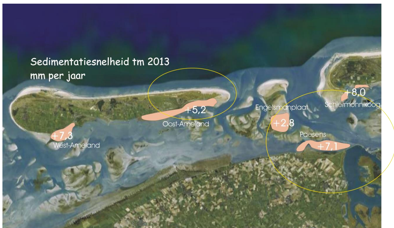
Figuur 24. Sedimentatiesnelheid per onderzoeksgebied in mm/jaar. De reeksen waarop het gemiddelde is gebaseerd variëren in lengte van 7 tot 13 jaar maar ze zijn allemaal bijgewerkt tm 2013.
