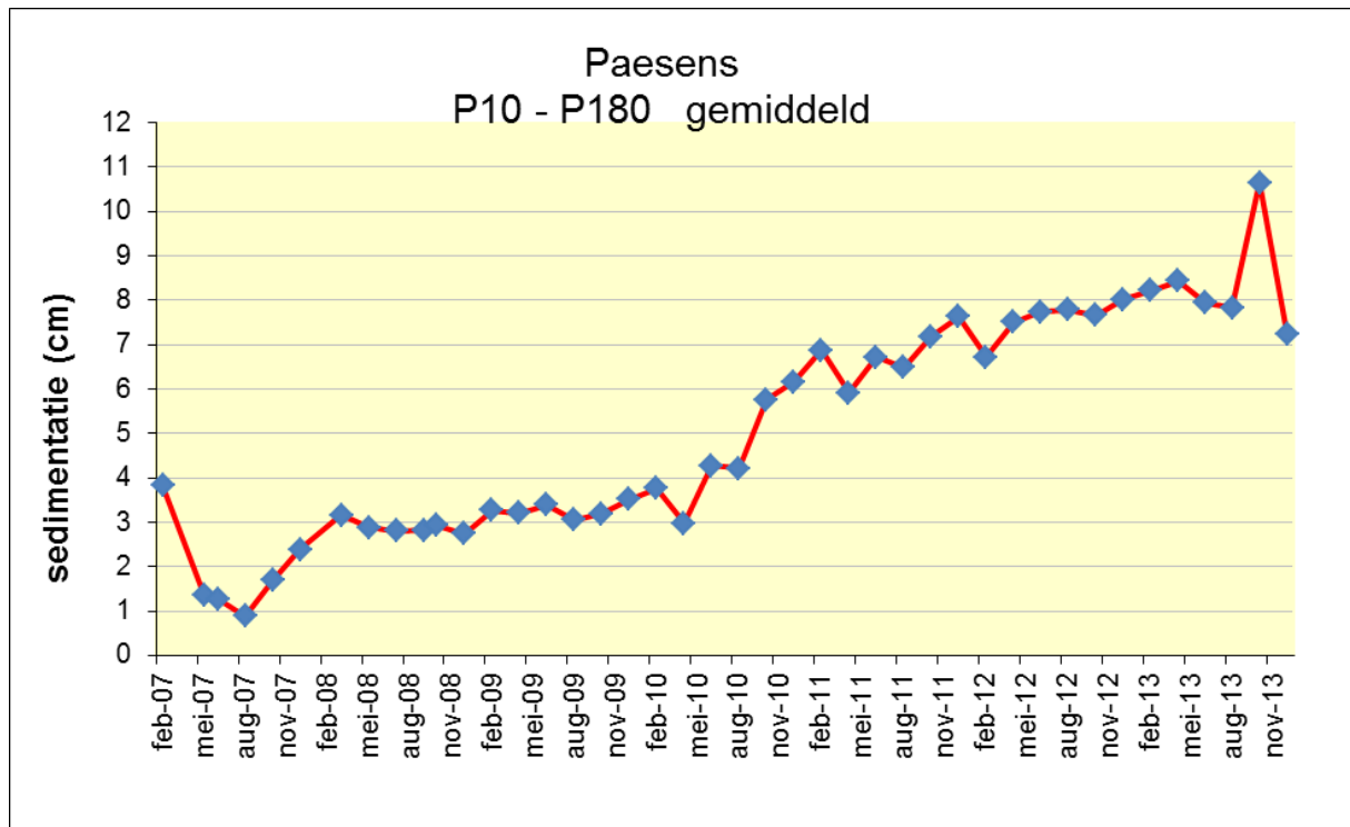
Figuur 15. Gemiddelde verschilmeting van de meetstations P10 tm P180 in het onderzoeksgebied bij Paesens.
