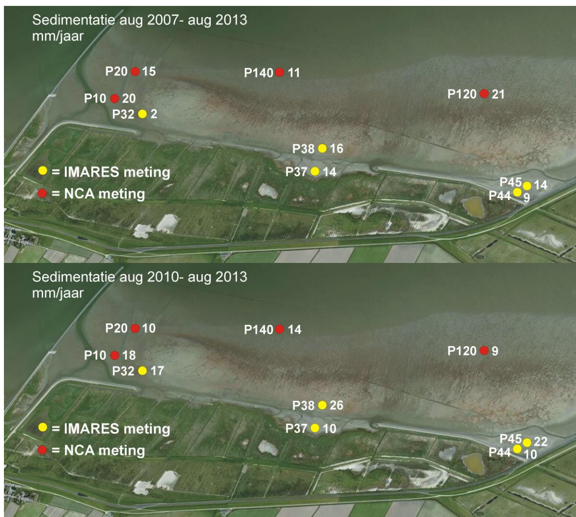
Figuur 33. Kaartbeeld met sedimentatie vergelijking van de meting van NCA en IMARES. Boven over periode aug2007-aug2013. Onder over periode aug2010-aug2013. Rechts van de gekleurde stip waarmee de locatie van het meetstation wordt aangeduid staat de sedimentatie in mm/jaar.
