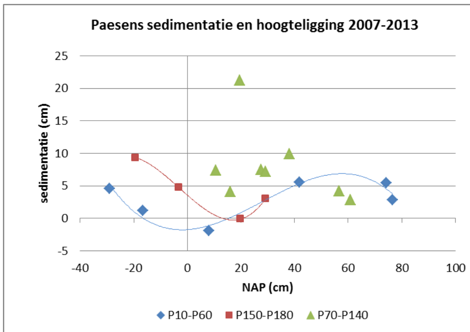
Figuur 30. Hoogteligging en sedimentatie van meetstations bij Paesens in de periode 2007-2013.
