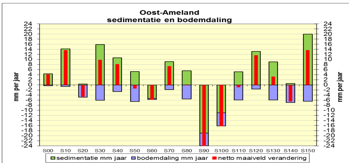
Figuur 31. Snelheid van sedimentatie en bodemdaling in mm/jaar gedurende de gehele meetperiode per meetstation (zie tabel 2). Bijgewerkt tm december 2011. De bodemdalingsnelheid is berekend tm 2010.
