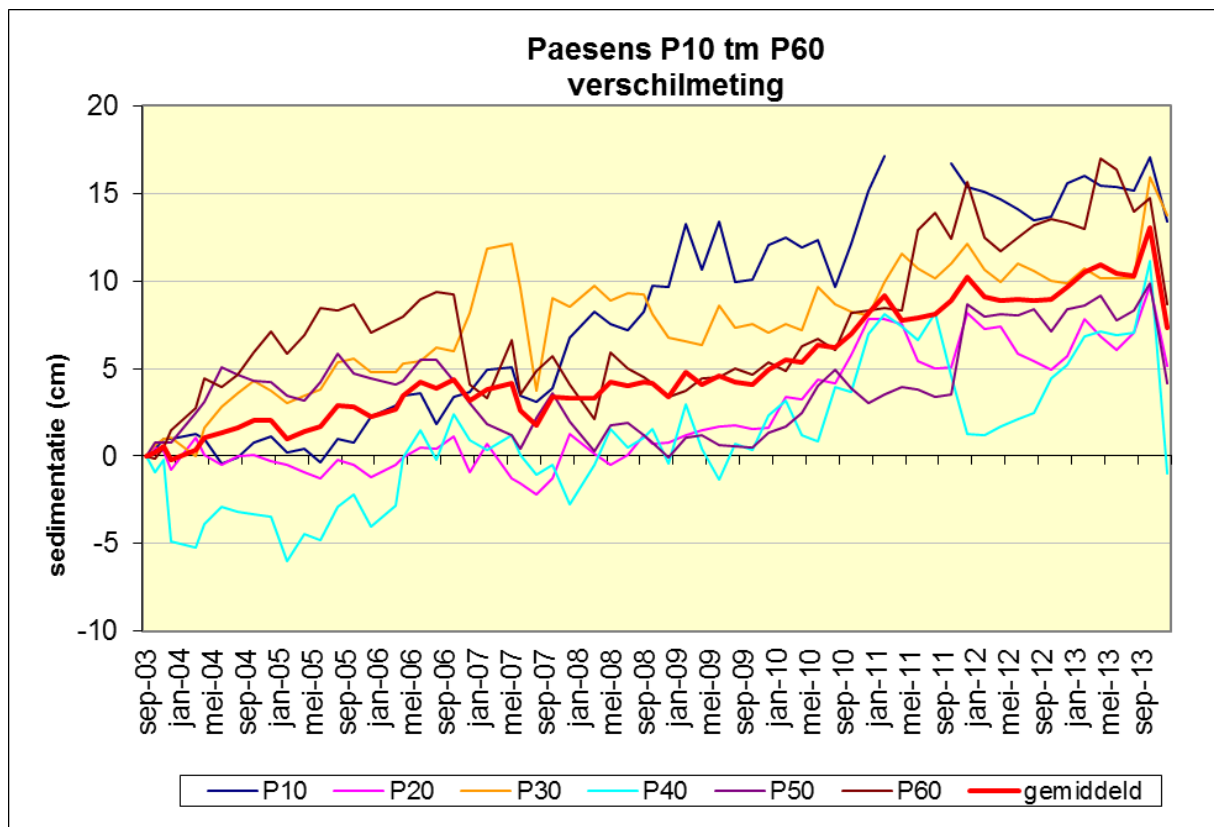
Figuur 13. Gemiddelde meetlijnen van de meetstations P10 tm P60 in het onderzoeksgebied bij Paesens. Tevens is het gemiddelde van deze 6 meetlijnen genomen als weergave van de sedimentatie van het gebied waarin de meetstations liggen.
