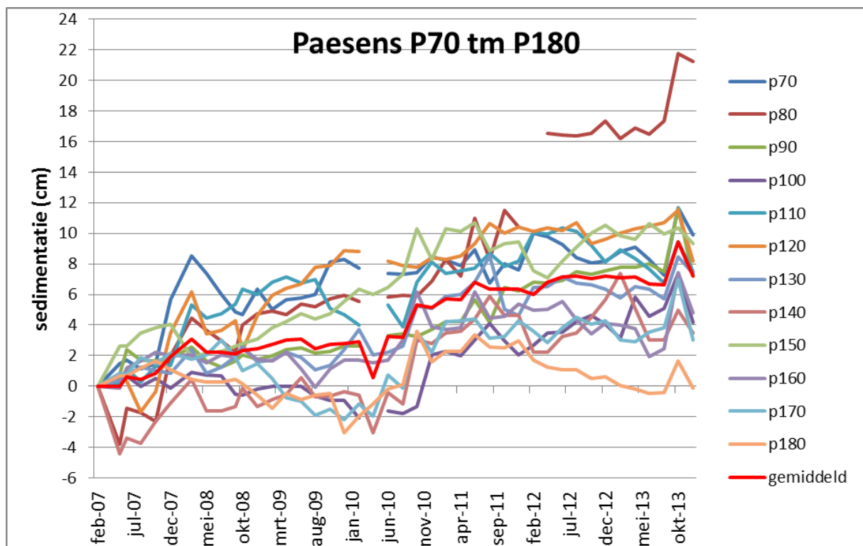
Figuur 14. Gemiddelde meetlijnen van de meetstations P70 tm P180 in het onderzoeksgebied bij Paesens. Tevens is het gemiddelde van deze 12 meetlijnen genomen als weergave van de sedimentatie van het gebied waarin de meetstations liggen.
