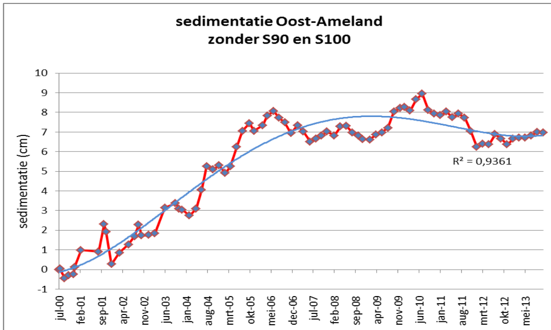
Figuur 21. Verschilmeting per keer en cumulatie van de meetstations S00 tm S180 (zonder S90 en S100) in het onderzoeksgebied Oost-Ameland.
