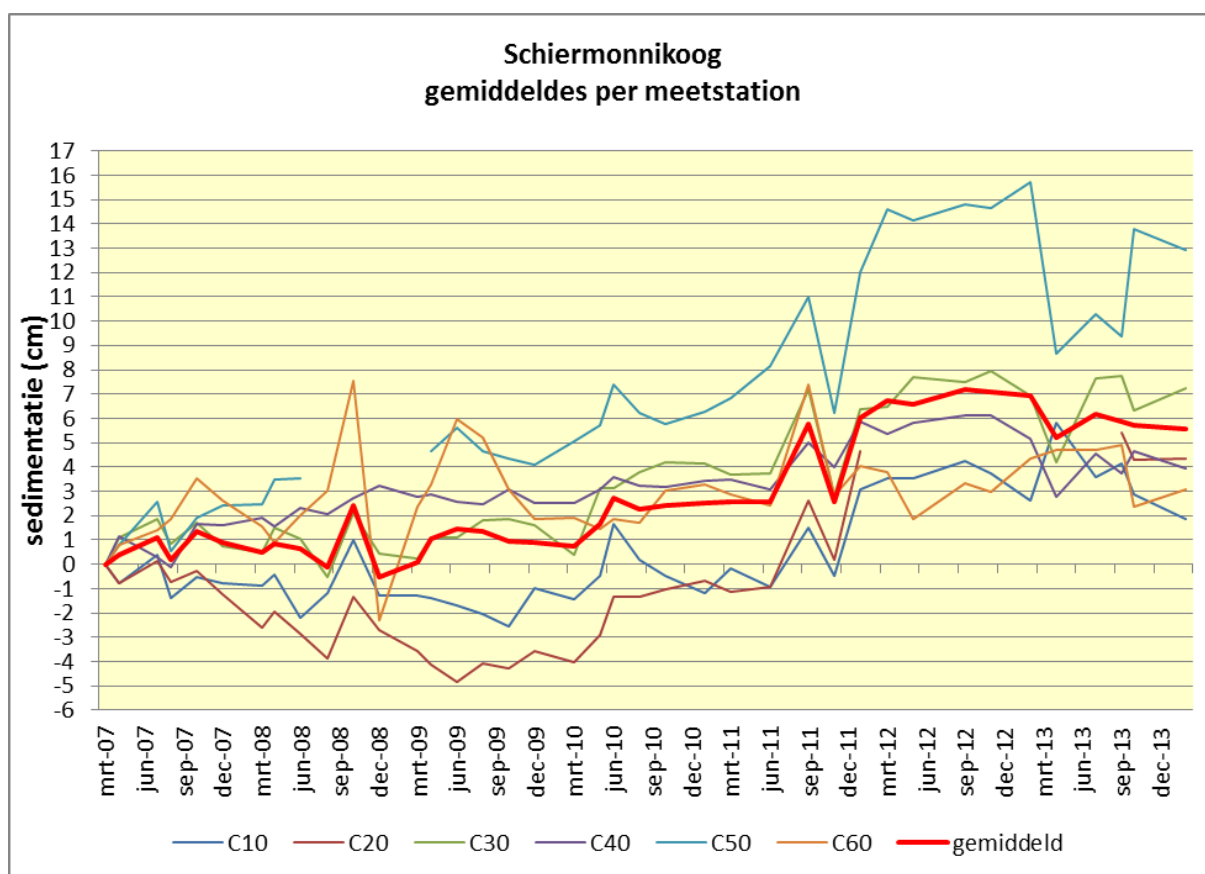
Figuur 18. Gemiddelde meetlijnen van de meetstations C10 tm C60 in het onderzoeksgebied Schiermonnikoog. Tevens is het gemiddelde van deze 6 meetlijnen genomen als weergave van de sedimentatie van het gebied waarin de meetstations liggen.
