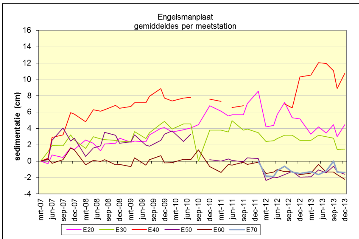
Figuur 16. Gemiddelde meetlijnen van de meetstations E10 tm E60 in het onderzoeksgebied Engelsmanplaat.
