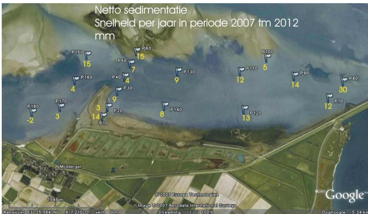
Figuur 32. Netto sedimentatie in millimeters per jaar in de periode 2007 tm 2012. Netto betekent dat de diepe daling van de sedimentatie is afgetrokken. Andere compenserende of versterkende factoren zoals zeespiegelstijging zijn niet verwerkt.
