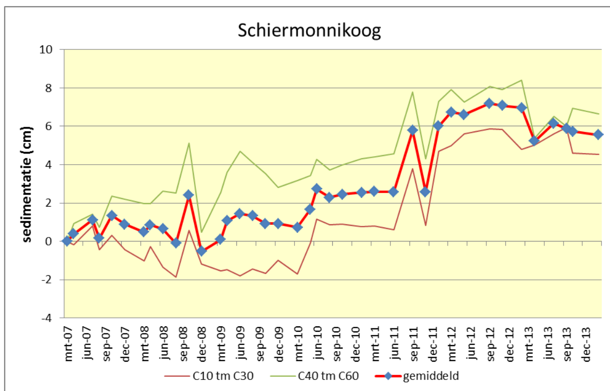
Figuur 19. Gemiddelde van de gebieden C10 – C30 (oost) en C40 – C60 (west) en het overall gemiddelde van de meetstations C10 tm C60 in het onderzoeksgebied Schiermonnikoog.
