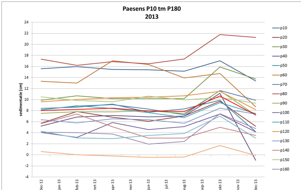
Figuur 35. Sedimentatie in 2013 van de stations P10 tm P180 in het onderzoeksgebied bij Paesens. De invloed van de stormen van 28 oktober (sedimentatie) en 5-6 december (erosie) is op alle 18 stations hetzelfde.
