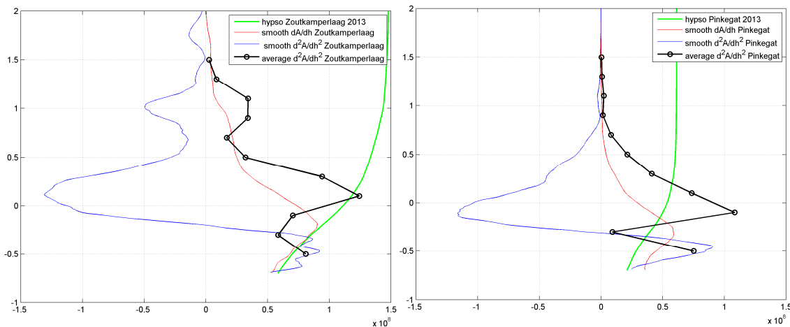
Figuur 5.3 Hypsometrische curve (groen) met eerste (rood) en tweede afgeleide (blauw). Op de horizontale as de oppervlakte [m²] en op de verticale as bodemhoogte [m NAP]. Afgeleiden zijn "gesmooth" met een window van 0.2 m. Zwarte lijn betreft de absolute waarde van het gemiddelde van de tweede afgeleide op het betreffende interval van de histogram.
