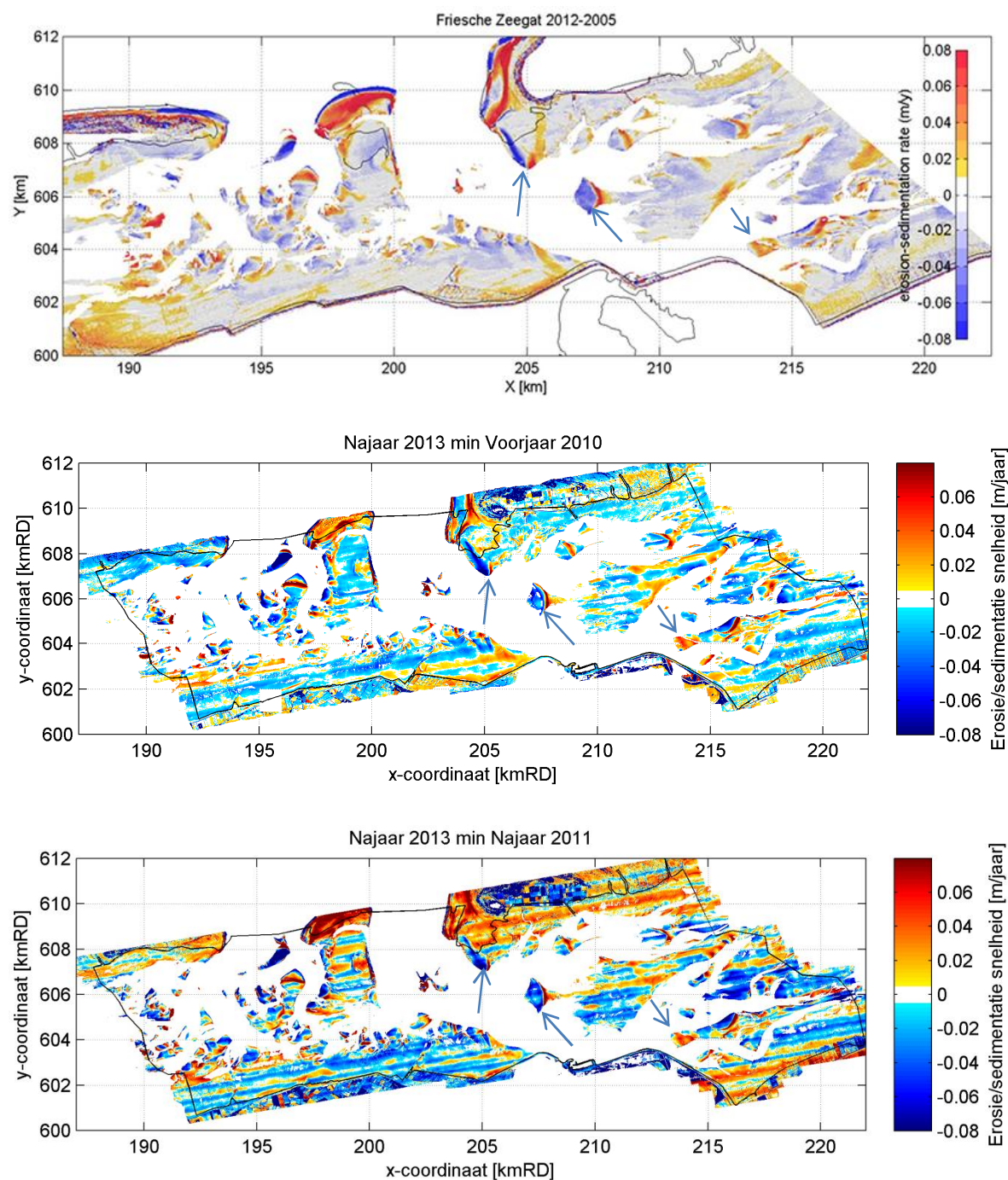
Figuur 4.5 Snelheid van sedimentatie (positief) en erosie (negatief) in m/jaar op basis van RWS vaklodingen voor de periode 2005-2012 (boven) en voor de LiDAR 2013 najaar minus 2010 voorjaar (midden) en LiDAR 2013 najaar minus 2011 najaar (onder).
