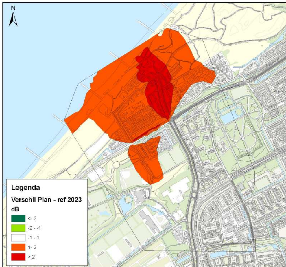
figuur 14.4 Verschilplot wegverkeerslawai plan 2023 -referentiesituatie 2023
