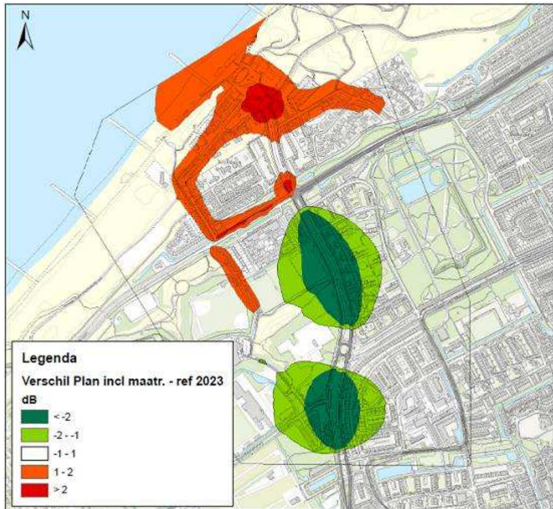
figuur 14.6 Verschilplot wegverkeerslawaa plan 2023 -referentiesituatie 2023
