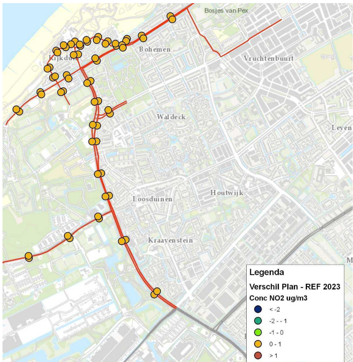
figuur 7.3 Verschil in jaargemiddelde concentratie \text{NO}_2 tussen het Voornemen en de referentiesituatie
