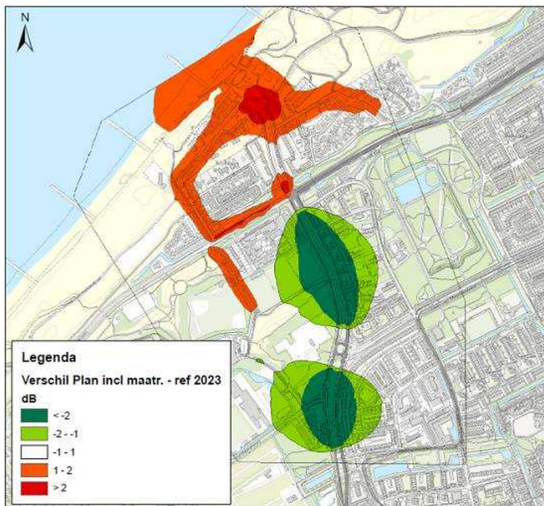
figuur 6.6 Verschilplot wegverkeerslawaai plan 2023 inclusief maatregelen - referentie 2023
