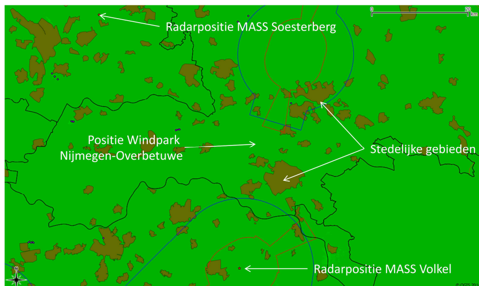
Figuur 5 Detectiekans van het MASS primaire verkeersleidingsradarnetwerk op 1000 voet boven het bouwplan voordat dit is gerealiseerd (baseline). De detectiekans is overall in het figuur 100% (donkergroen). Op dit figuur is detectiekansmiddeling toegepast.
