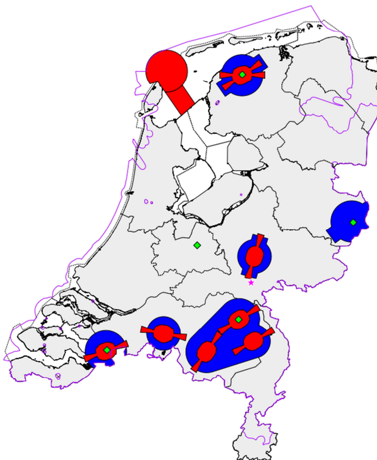
Figuur 4. De ligging van het te toetsen bouwplan aangegeven met een ster en de ligging van de thans gehanteerde 2014-2 normhoogtes op 300 voet (rood) en 500 voet (blauw). Op 1000 voet (paars) dient het MASS radarnetwerk, op enkele uitzonderingen na, een landelijke dekking te hebben. Tevens zijn op deze kaart met een groene markering de locaties aangegeven van het MASS verkeersleidingsradarnetwerk bestaande uit een vijftal radarsystemen.
