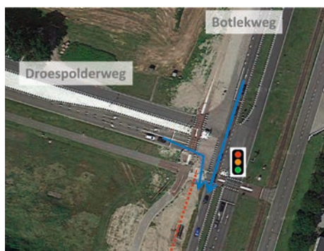
3 Verdubbelen Botlekweg, rechtsaf vanaf Droespolderweg en doorgaand op Botlekweg gelijktijdig groen licht geven
