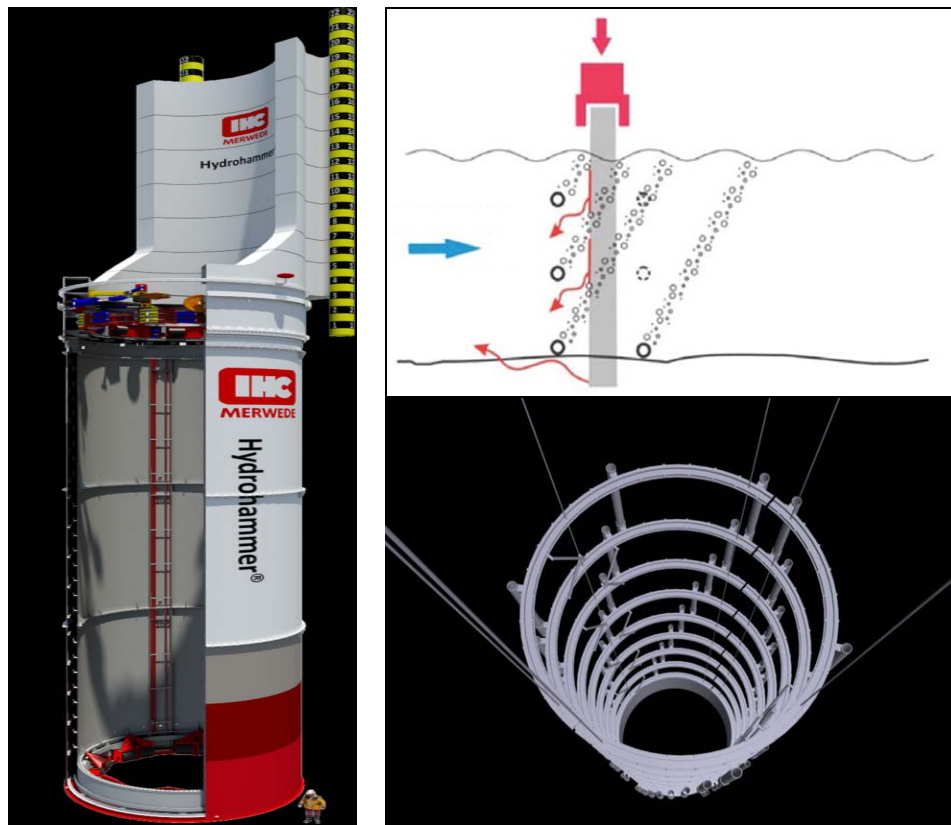
Dubbelwandige cilinder Bellenscherm Figuur 9: mogelijke technieken om de geluidsemisatie tijdens heiverkzaamheden te reduceren
