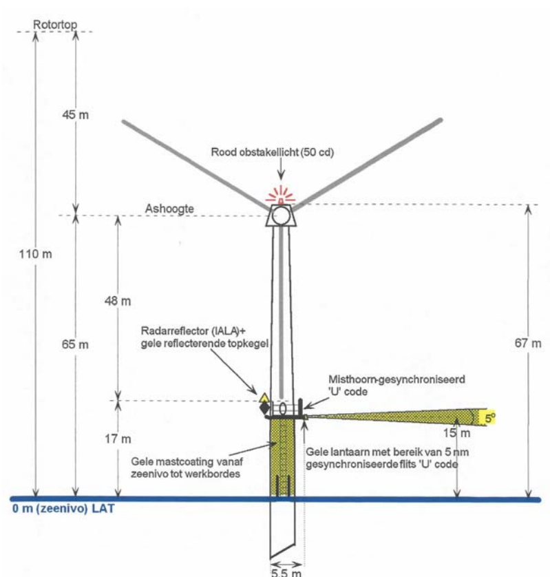
Figuur 13: Verlichting windturbine voor luchtvaart en scheepvaart 27
