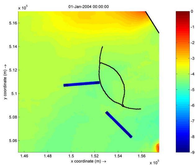
Figuur 2.9: Scenario Variant 2b - Kenmerken: 2 geulen: 3,1 km, Diepte geulen: 4 m t.o.v. omgeving, Uiteinden: 10 m t.o.v. omgeving, Vergraving: 7,3 miljoen m3
