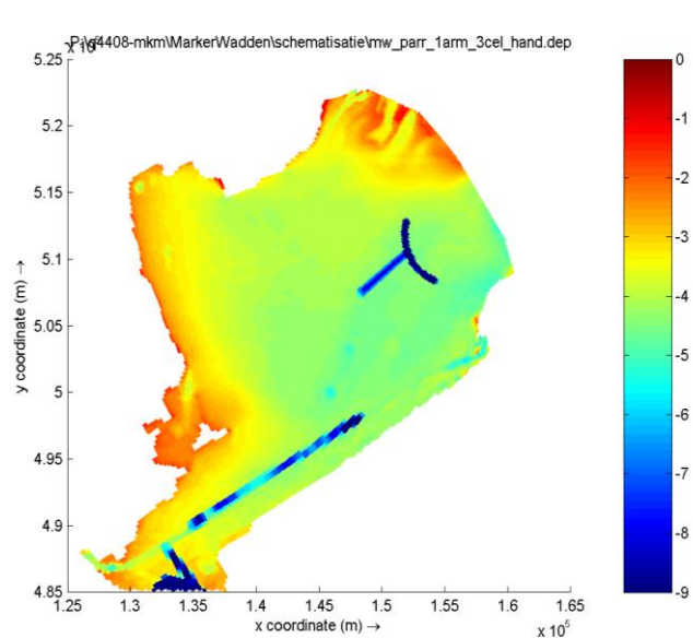
Figuur 2.2: Scenario MW03 - Kenmerken: Hoofdgeul: 5,9 km gekromd, 1 zijtak breed: 4,8 km, Vergraving: 19 miljoen m 3
