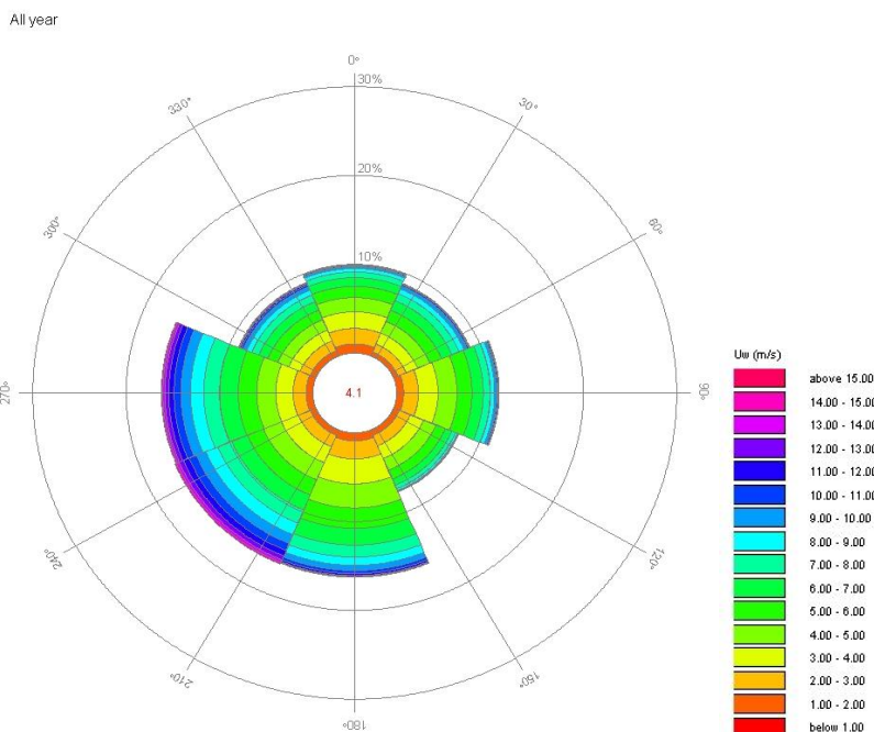
Figuur 3.8: Verdeling wind, periode 1951-2013
