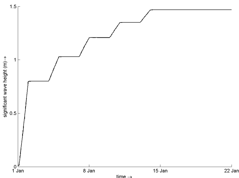
Figuur 3.9: Golfhoogteverloop (m) in de tijd voor een punt in het luvtegebied bij noordwestenwind
