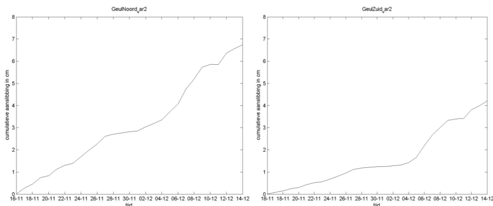
Figuur 3.4: Vergelijking aanslibbing in noordgeul (links) en zuidgeul (rechts) voor variant 2a in de periode 16 november tot 14 december
