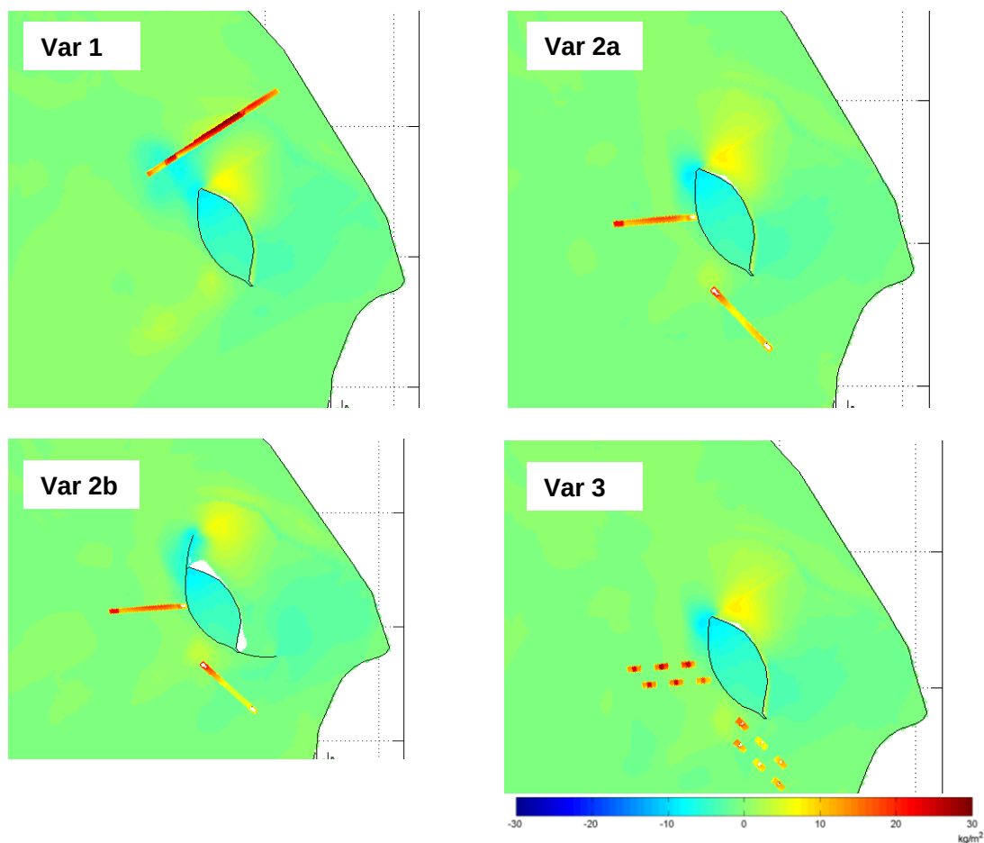
Figuur 3.5: Aanslibbing en erosie t.o.v. referentie situatie van de 2e set berekeningen. geel / oranje = sedimentatie, blauw = erosie. Eenheid is kg/m 2
