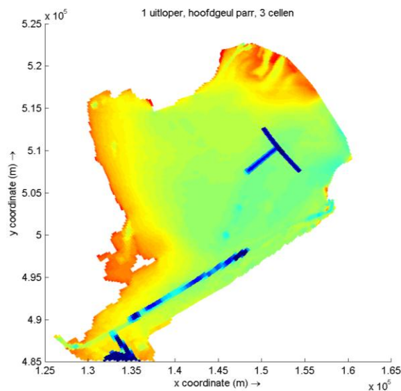
Figuur 2.3: Scenario MW04 - Kenmerken: Hoofdgeul: 6,7 km recht, 1 zijtak breed: 4,8 km, Vergraving: 18 miljoen m 3
