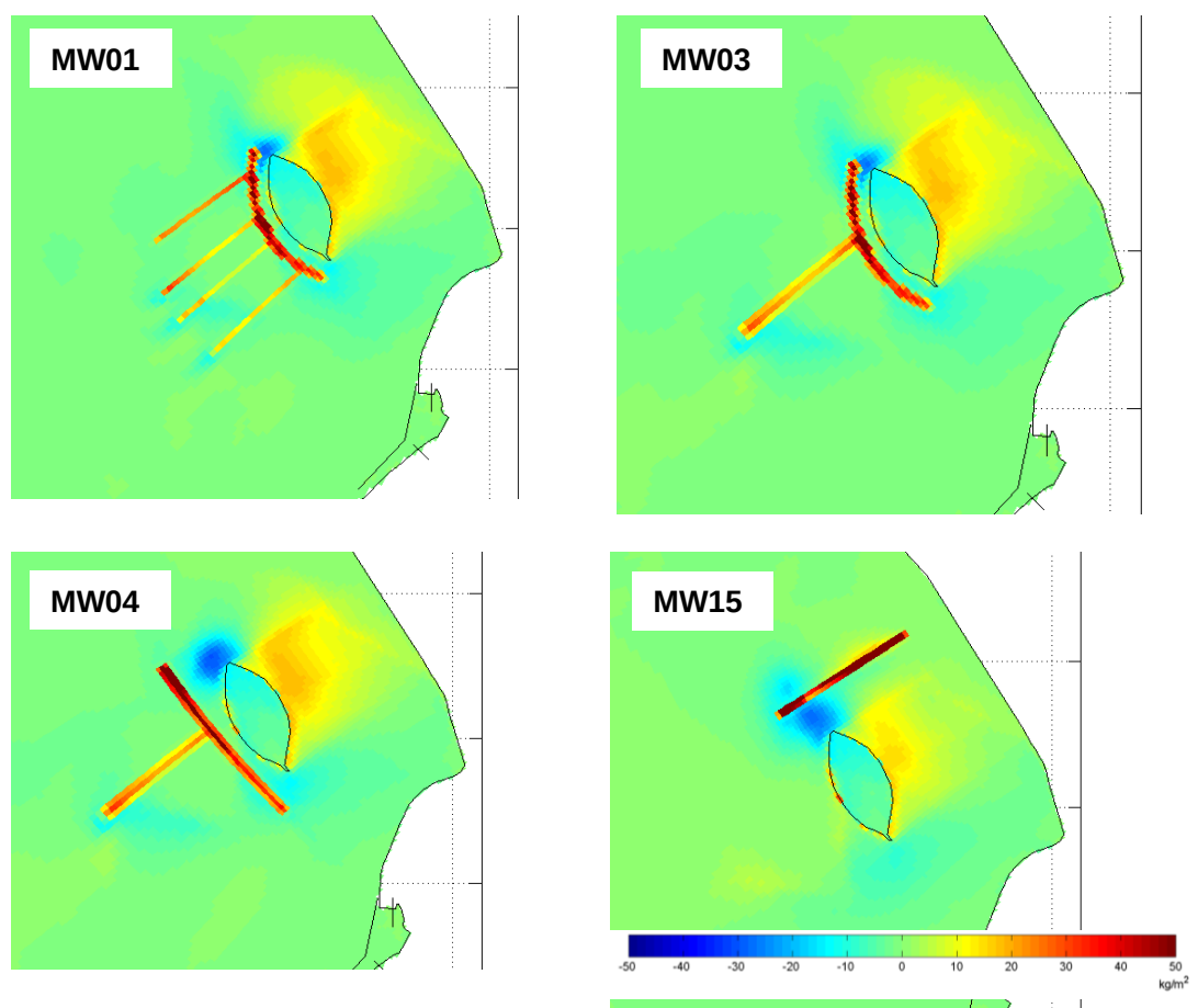
Figuur 3.1: Aanslibbing en erosie t.o.v. referentie situatie. geel / oranje = sedimentatie, blauw = erosie. Eenheid is kg/m 2
