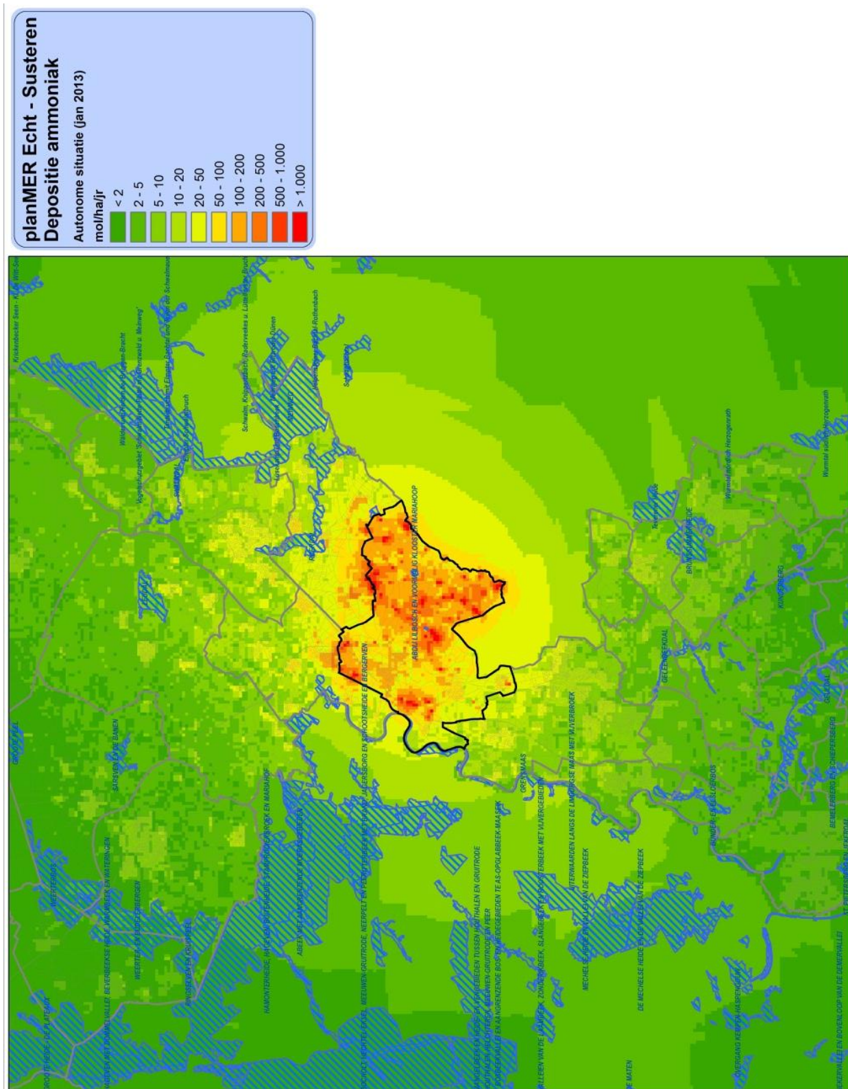
Gemeentelijke bijdrage aan de stikstofdepositie in de huidige situatie + autonome ontwikkeling (referentiesituatie) (zwarte lijn: gemeente Echt-Susteren, blauwe lijn: Natura 2000-gebieden)
