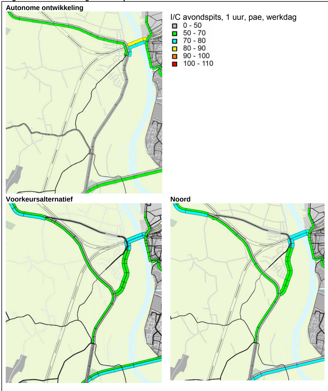
Figuur 6.6 I/C-verhoudingen avondspits in 2030
