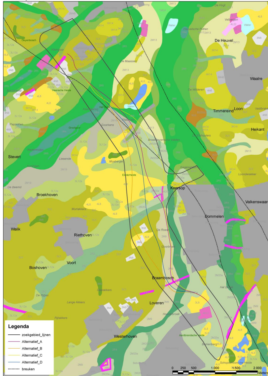
Geomorfologische kaart
