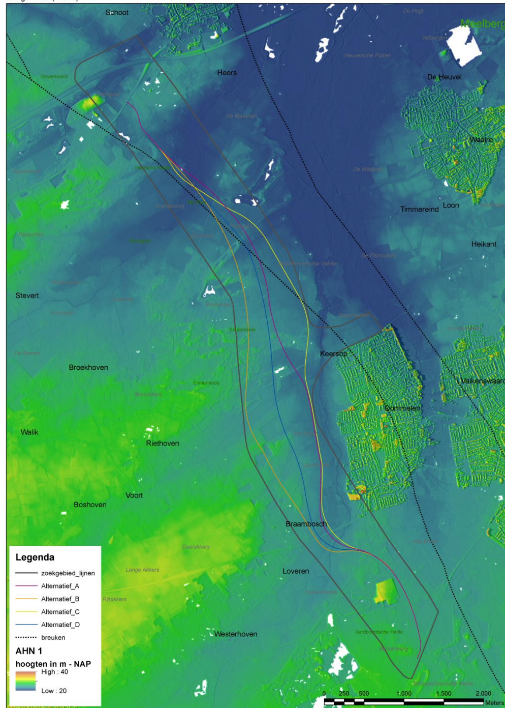
Hoogtekaart (AHN1)
