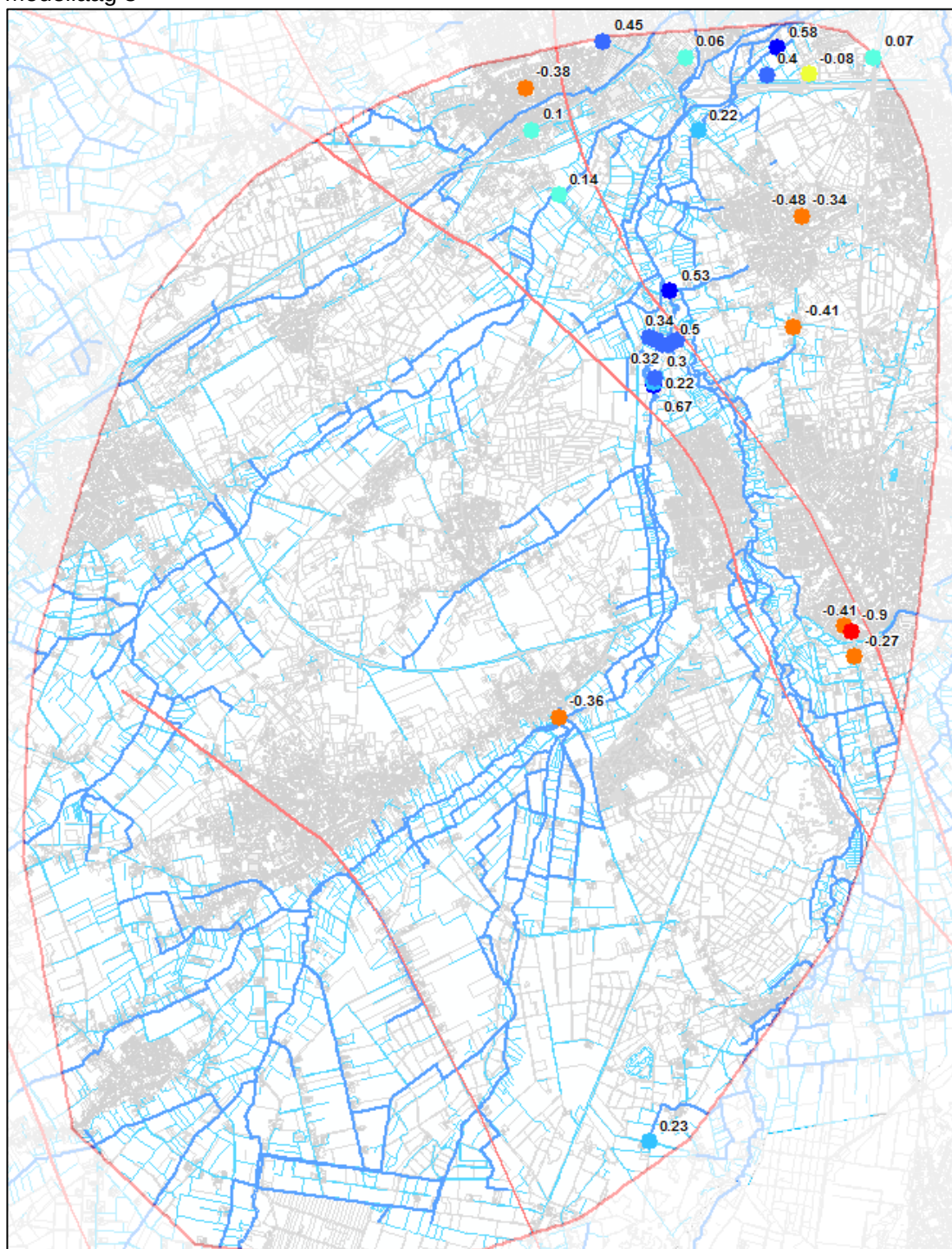
Modellaag 3
