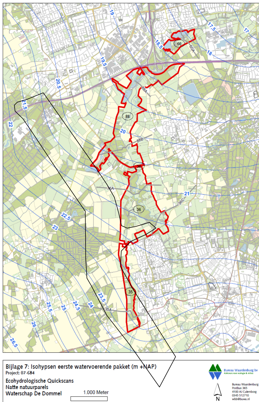
Figuur 4.8 Isohypsens (grondwaterdruk) in het eerste watervoerend pakket
