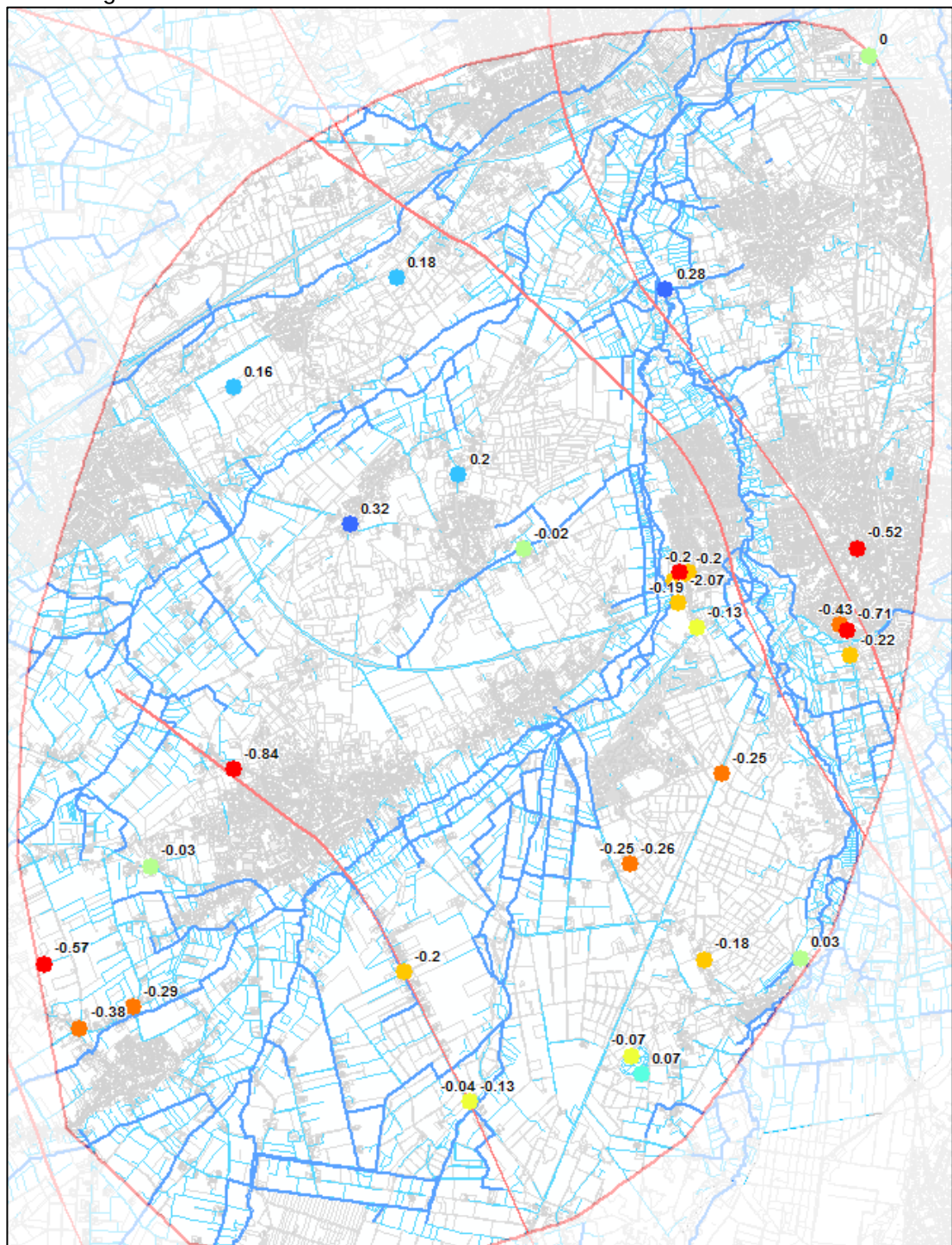
Modellaag 5
