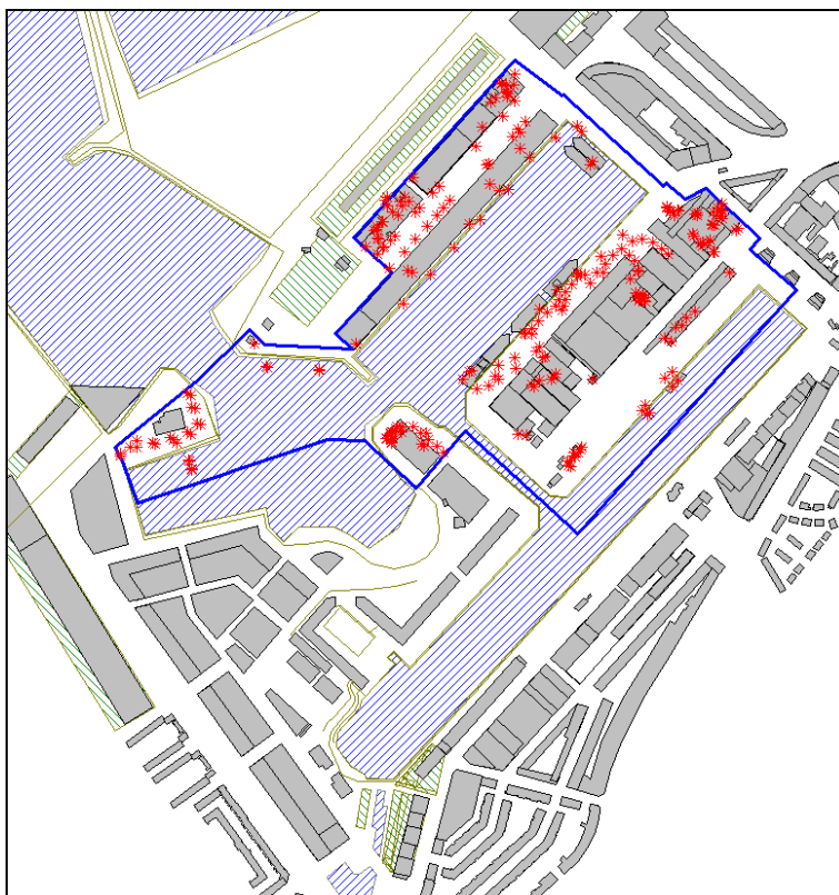
Figuur 7.1: Nieuwe gezoneerde Industrieterrein met aanwezige bronnen (VKA), situatie 2013
