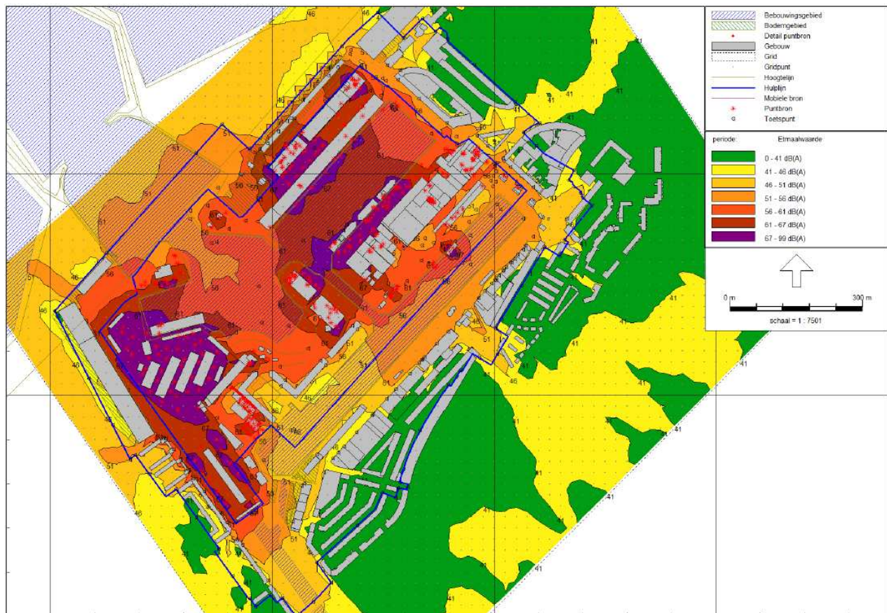
Figuur 5.2: Geluidcontouren geluidbelasting LA_{eq} industrielawaai, situatie 2006
