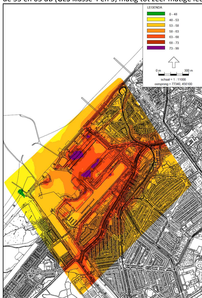
figuur 6.2 Gecumuleerde geluidbelasting referentiesituatie
