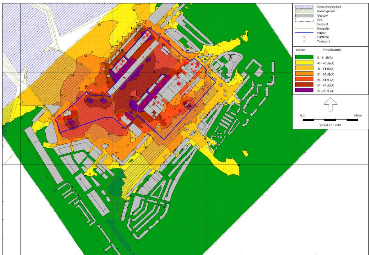
Figuur 8.1: Geluidcontouren geluidbelasting LA_{eq} industrielawaai, VKA met walstroom 2013
