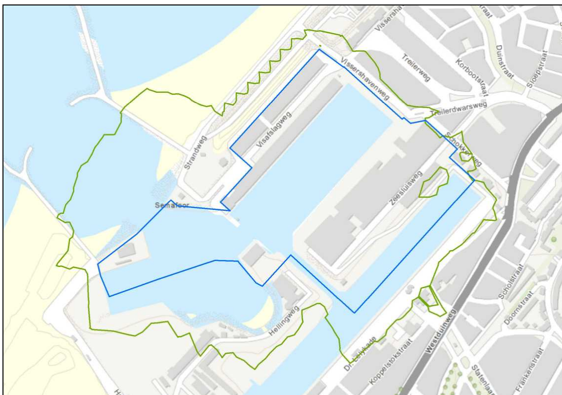
Figuur 12.2 51 dB(A)-contour op 5 meter hoogte (groene lijn) rondom het industrieterrein (blauwe lijn)
