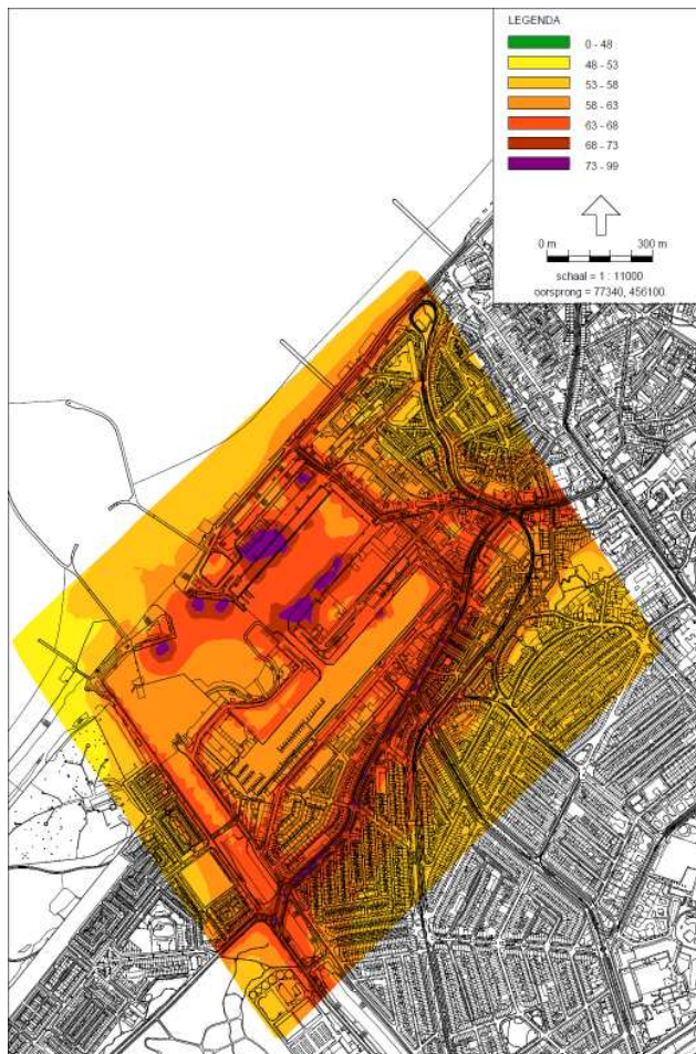
figuur 7.3 Gecumuleerde geluidbelasting voorkeursalternatief
