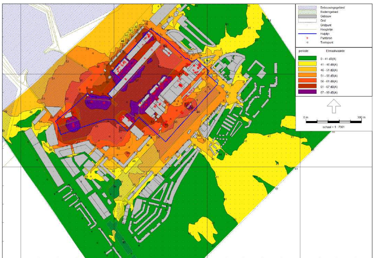
Figuur 7.2: Geluidcontouren geluidbelasting LA_{eq} industrielawaai, VKA 2013
