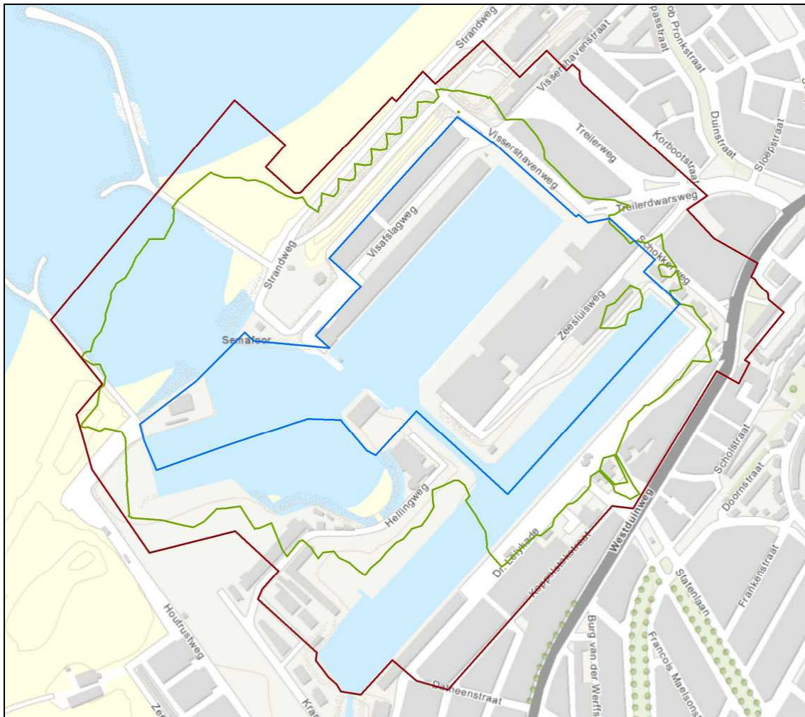
Figuur 12.3 Zonegrens (rode lijn) rondom de 51 dB(A)-contour op 5 meter hoogte (groene lijn)
