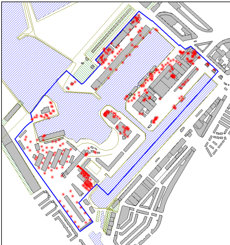
Figuur 5.1: Gezoneerde industrieterrein met aanwezige geluidbronnen, situatie 2006
