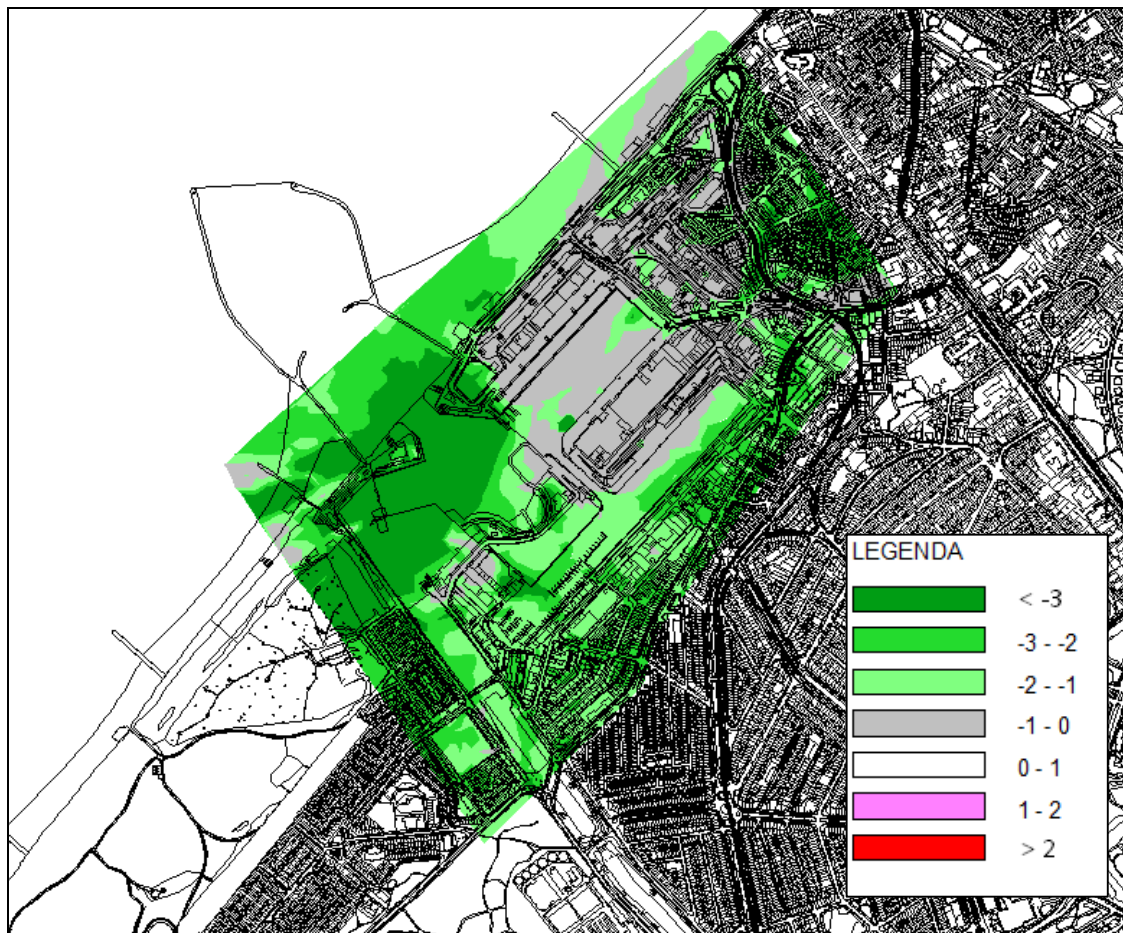
Figuur 8.2: Verschilplot VKA met walstroom 2013 - VKA zonder walstroom 2013 (waarden in dB)
