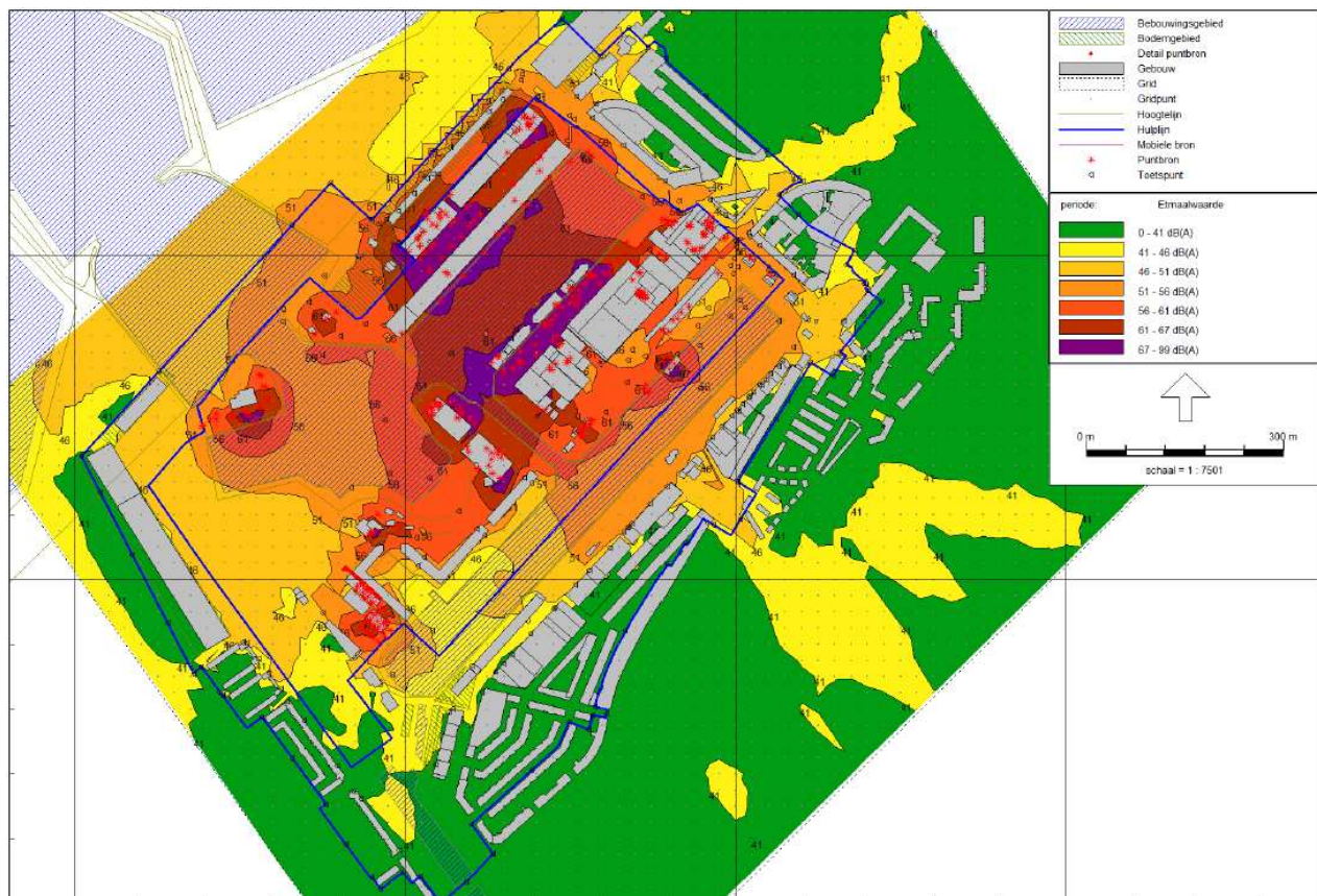
Figuur 6.1: Geluidcontouren geluidbelasting LA_{eq} industrielawaai, situatie 2013
