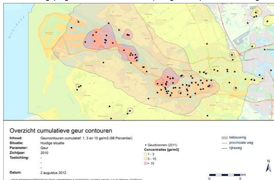
Figuur 5.9.1 Cumulatieve geurcontouren in de huidige situatie
