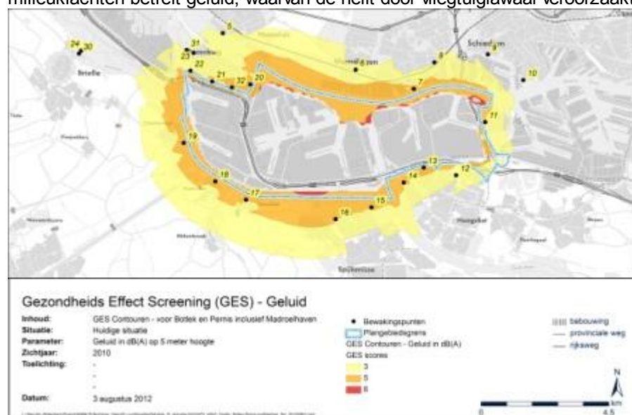
Figuur 5.10.1 Huidige Situatie: GES-kaart van geluid door industrie in de vergunde situatie voor deelgebied Botlek-Vondelingenplaat
