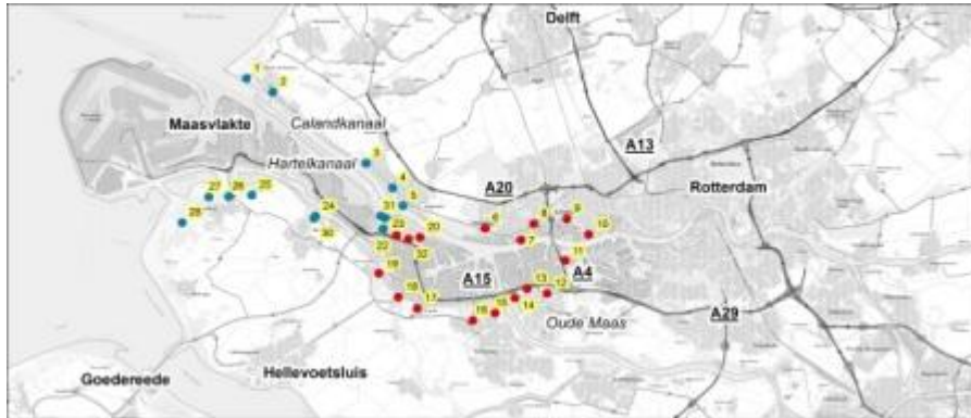
Figuur 5.3.1 Ligging referentiepunten (Zip) blauw = referentiepunten MV1/Europoort, rood = referentiepunten Botlek-Vondelingenplaat
