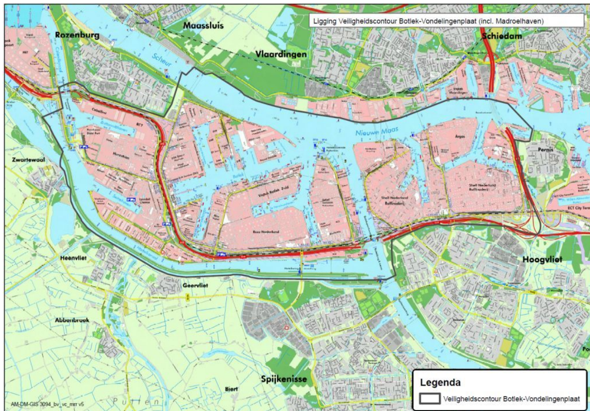
Figuur 4.4 Ligging Veiligheidscontour Botlek-Vondelingenplaat
