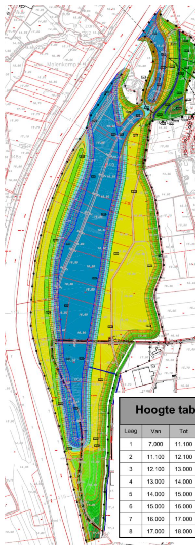
Figuur 5: globaal ontwerp geoptimaliseerde hoogwatergeul (exclusief kassengebied) en dwarsprofiel
