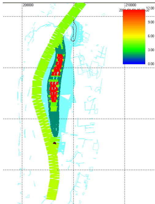
Figuur 4: Ontwerp DUFLOW met diepteverdeling met een maximale helderheid,
