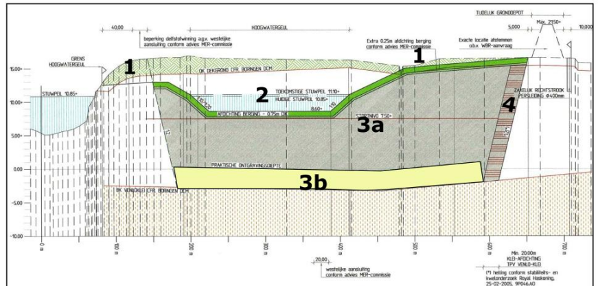
Dwarsprofiel oorspronkelijke situatie
