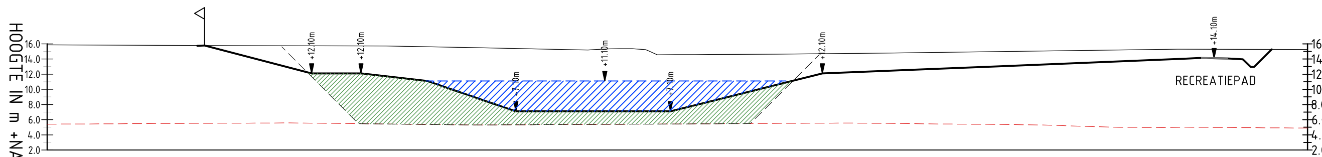
DWARSPROFIEL 8
