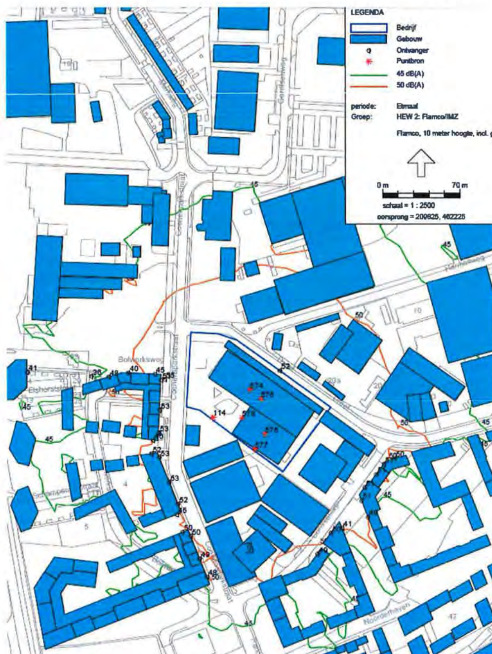
Figuur 25. Industrielawaai - IL, Zonebeheermodel Zutphen - versie van Zonebeheermodel Zutphen - Flamco, 45 en 50 dB(A)-etmaalwaardecontour op 10 meter boven maaiveld, inclusief bestaande bebouwing en nieuwbouw Noorderhaven, geluidsbronnen volgens zonebeheermodel (gemeente Zutphen)
