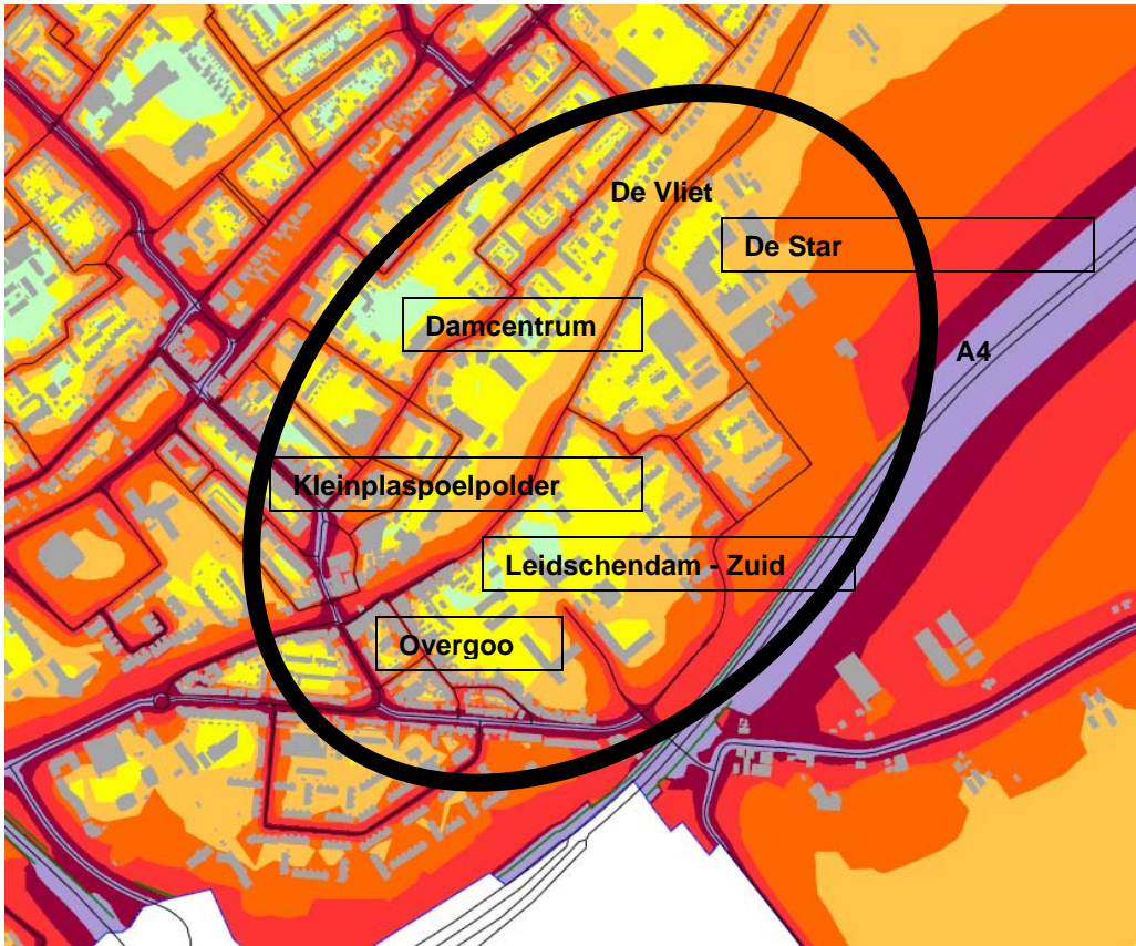
Uitsnede contourenkaart wegverkeer, gebied rond opgave Leidschendam - Centrum
