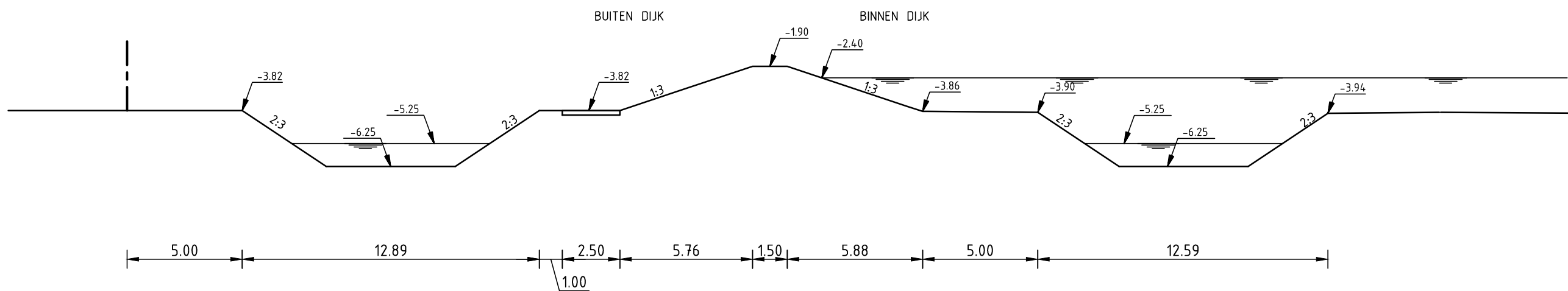
Dwarsprofiel 1 Noordzijde Schaal 1:200
