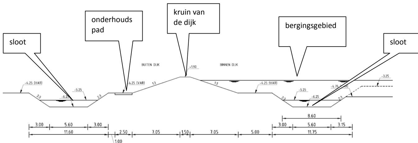
Principe profiel ringdijk piekberging
