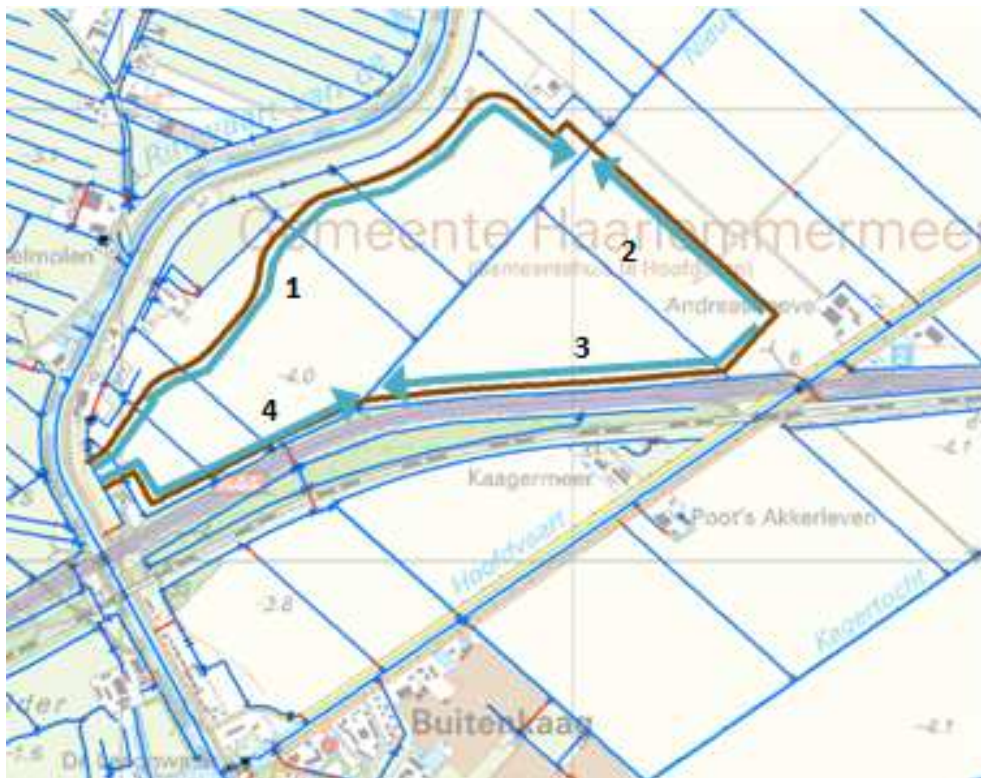
Figuur 5.9: Werking watersysteem binnenzijde piekberging.
