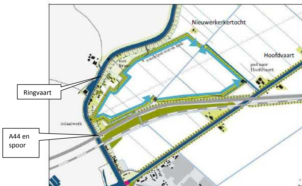
Figuur 5.3: Alternatief 1 'Laag en groot' [van Paridon x de Groot, 2011]
