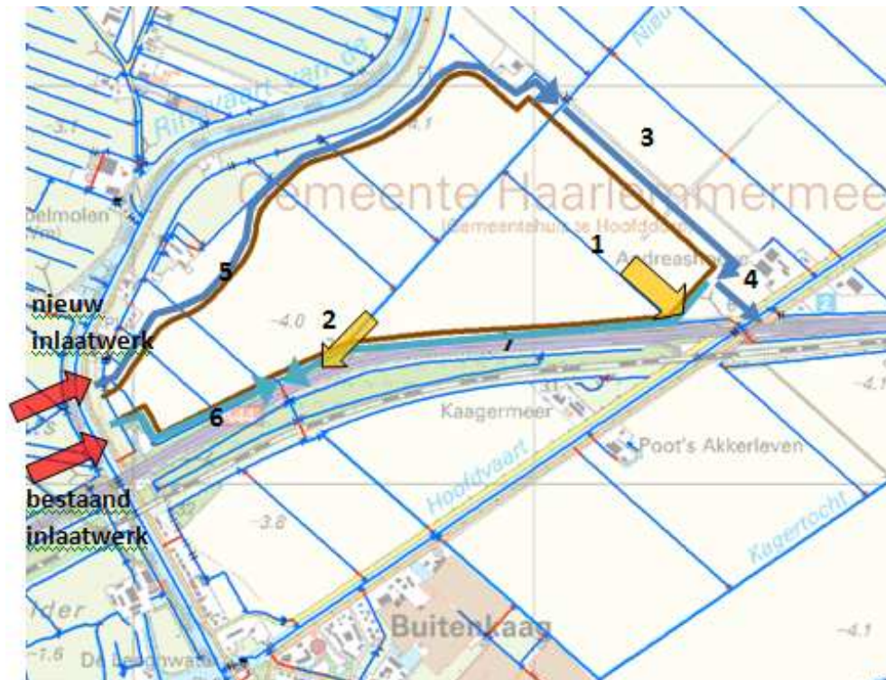
Figuur 5.8: Werking watersysteem buitenzijde piekberging.
