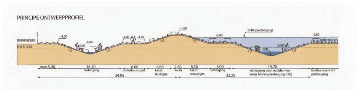
Figuur 4.3: Principe ontwerp-profiel.
