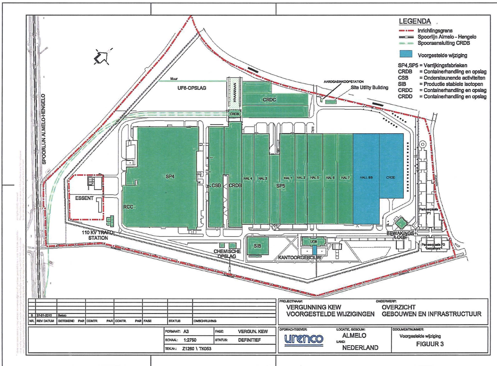
Fig. 3 Eindsituatie 6.200 tSW/jaar
