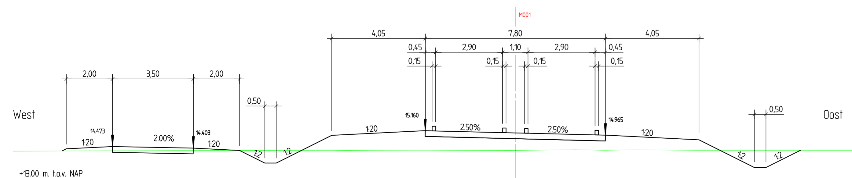
Dwarsprofiel 1-1 Meetring : 100.000 rijbaan + incl. bochtverbreiding schaal 1:100
