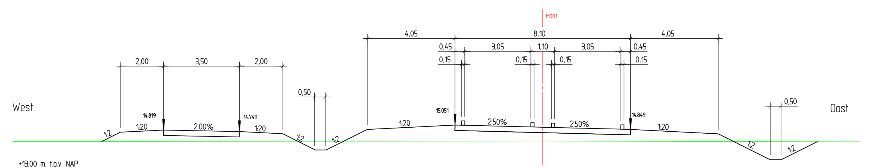
Dwarsprofiel 9-9 Metrening : 2350.000 rijbaan = incl. bochtverbredening schaal 1:100
