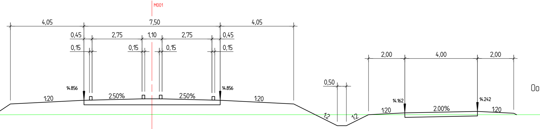
Dwarsprofiel 6-6 Metering: 1:50.000 schaal 1:100
