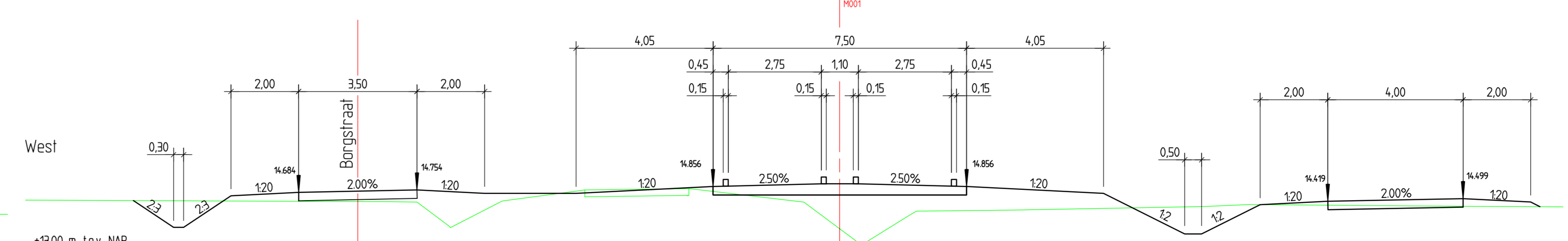
Dwarsprofiel 6-6 Metering: 1:50.000 schaal 1:100
