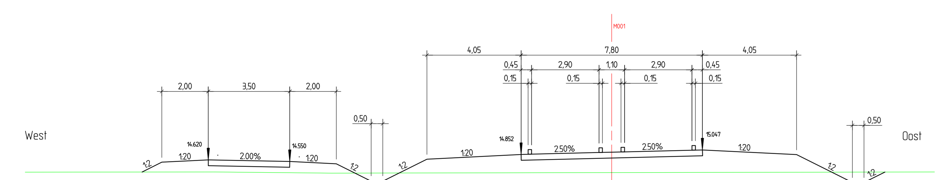
Dwarsprofiel 8-8 Metrening : 2200.000 rijbaan = incl. bochtverbredening schaal 1:100
