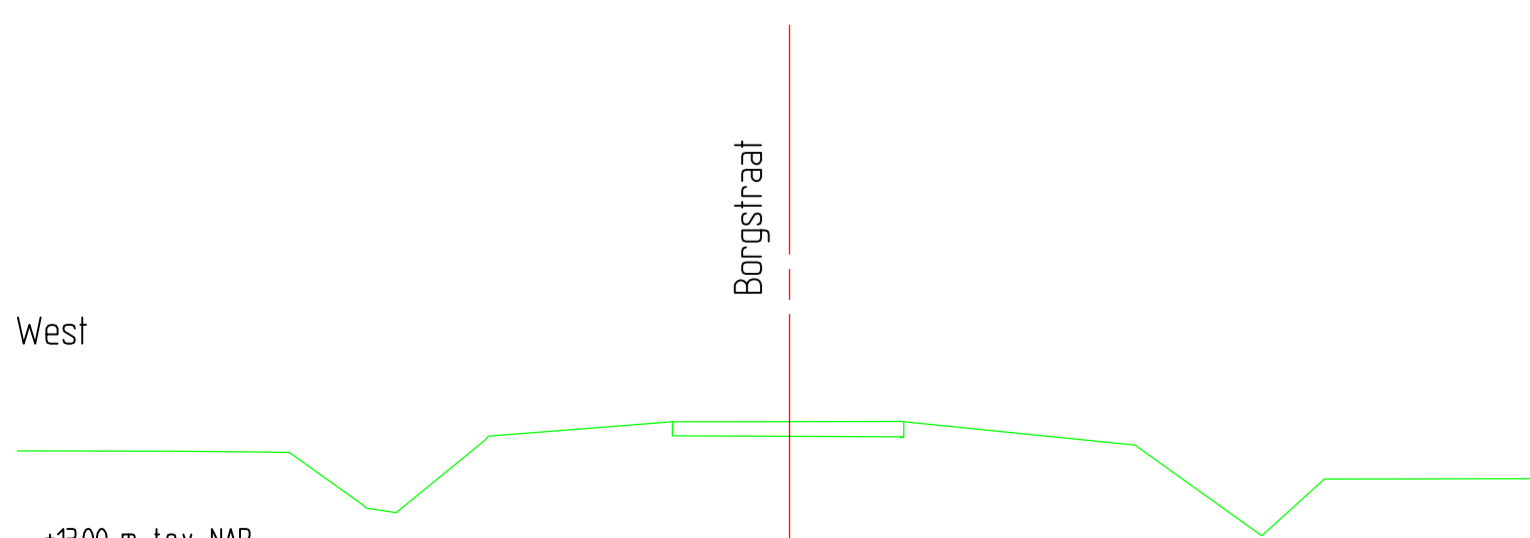
Dwarsprofiel 5-5 Metering: 1:100.000 schaal 1:100
