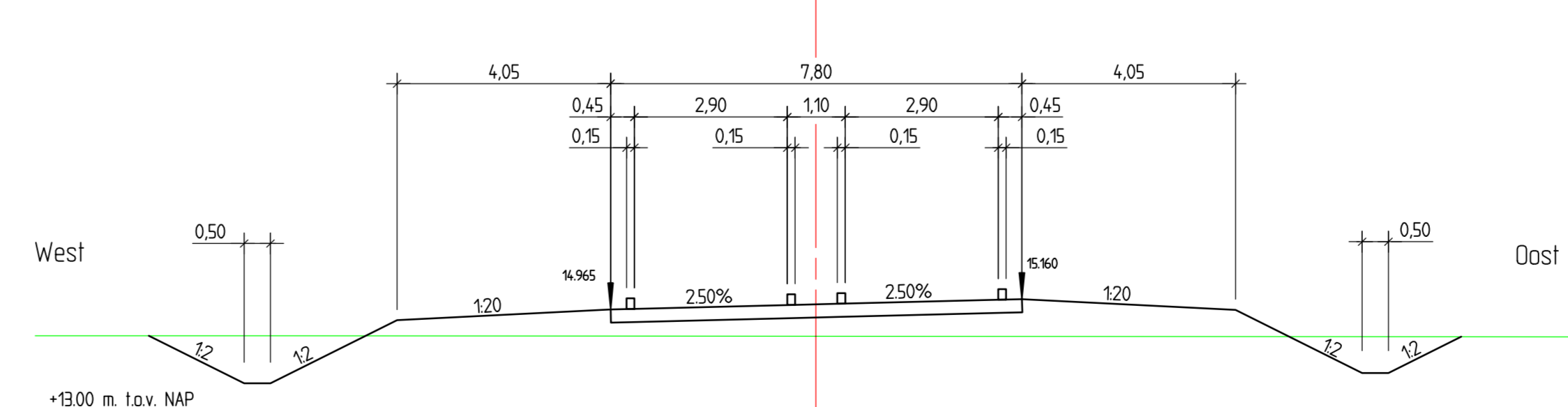
Dwarsprofiel 2-2 Meetring : 300.000 rijbaan + incl. bochtverbreiding schaal 1:100
