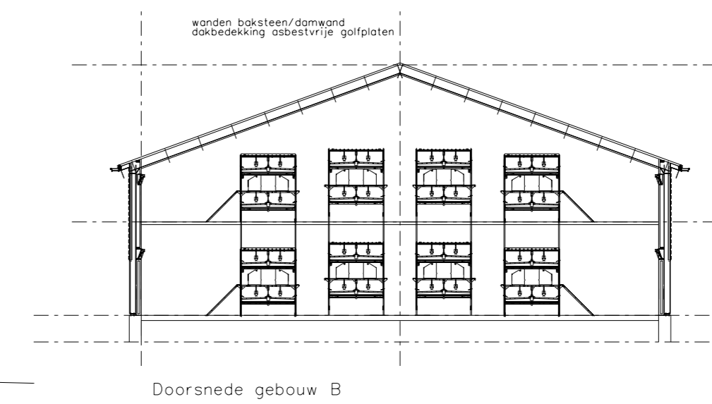
Doorsnede gebouw B
