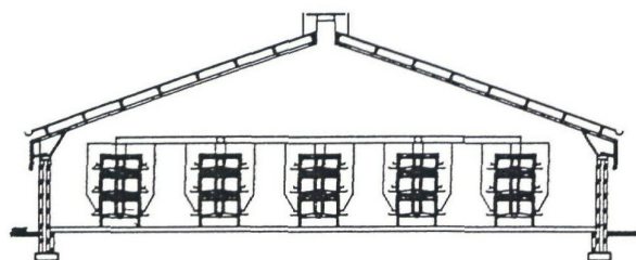
Dwarsdoorsnede
