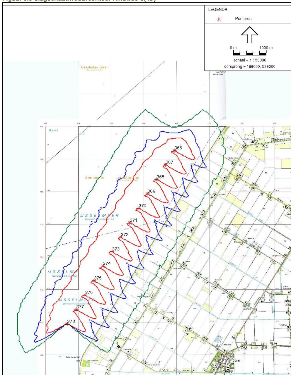
Figuur 5.5 Slagschaduwduurcontour NMDbu5-8(4D)
