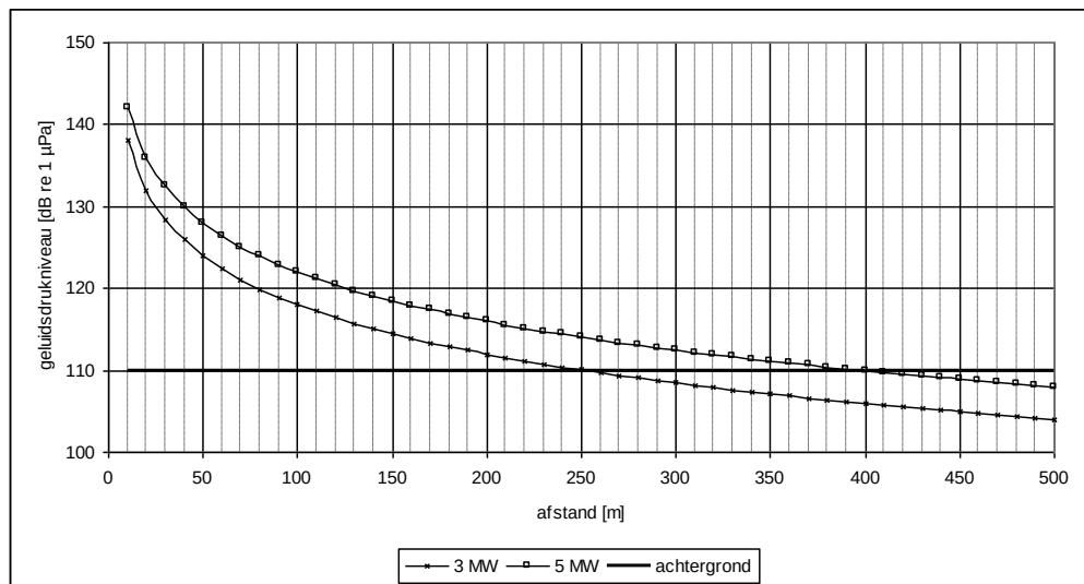
Figuur 5.4 Geluidsdruk niveau onder water op diverse afstanden
