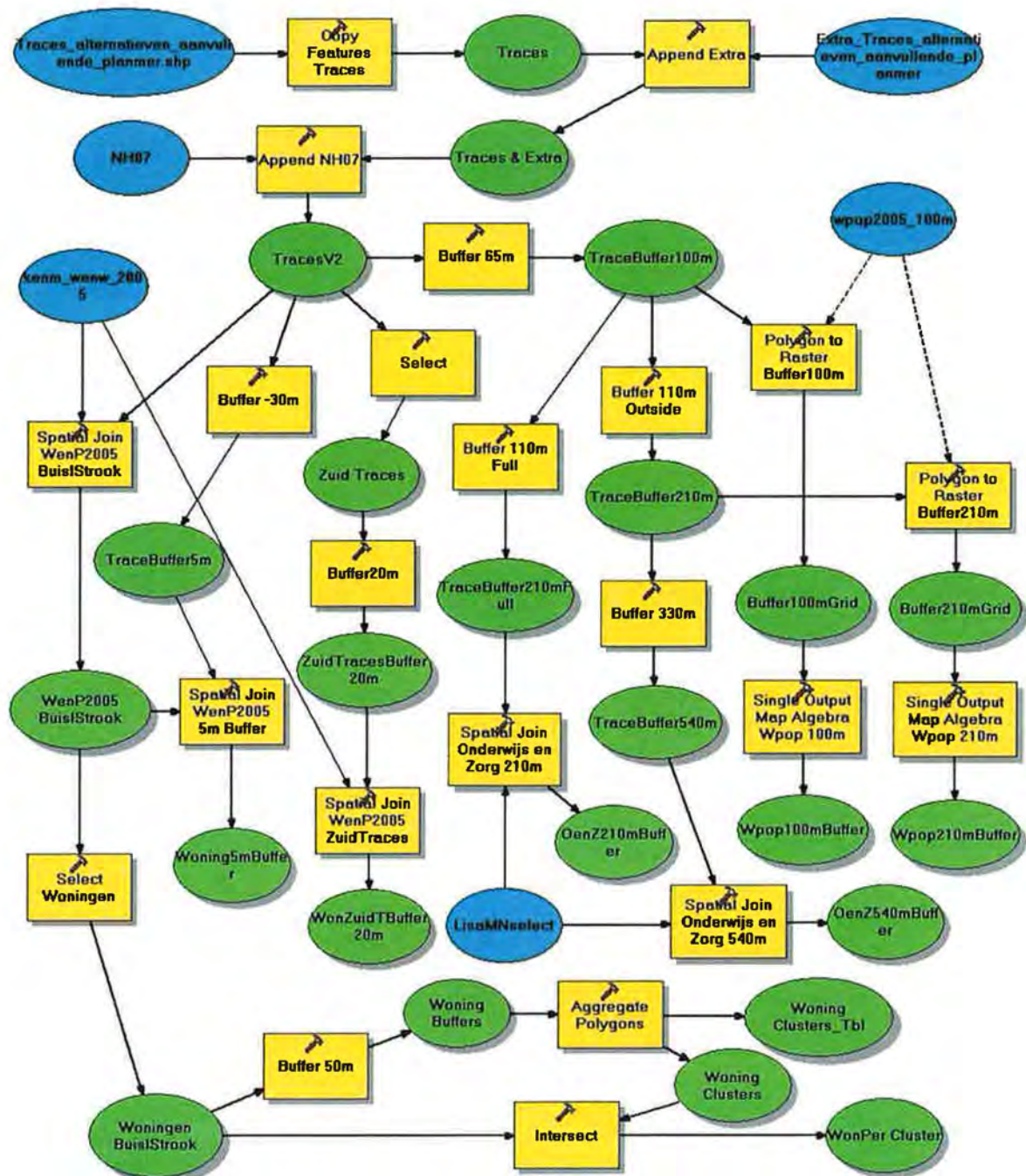
Figuur 3: Modelbuilder model voor de GIS-analyses van de 78 alternatieven
