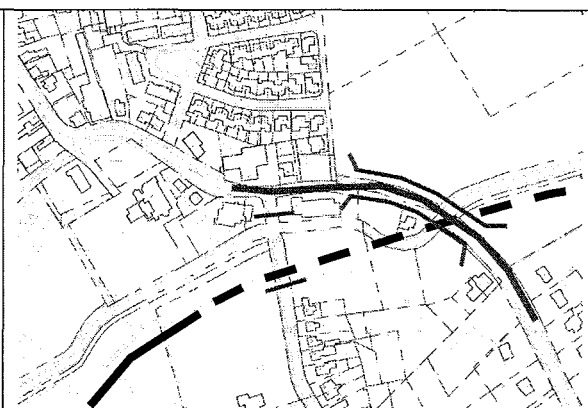
Figuur 4: Randweg in tunnelbak met ongelijkvloerse kruising bij de Kapellekestraat
