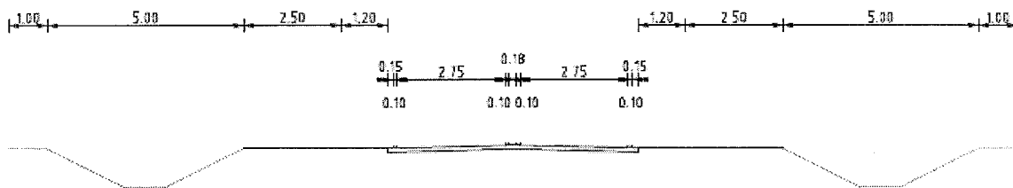
Profiel 50km/uur
