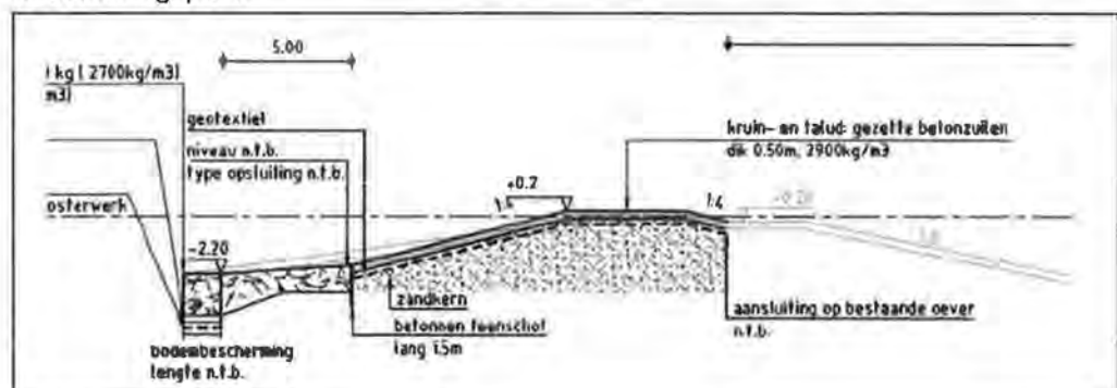
Dwarsdoorsnede Nieuw Uitwateringskanaal
