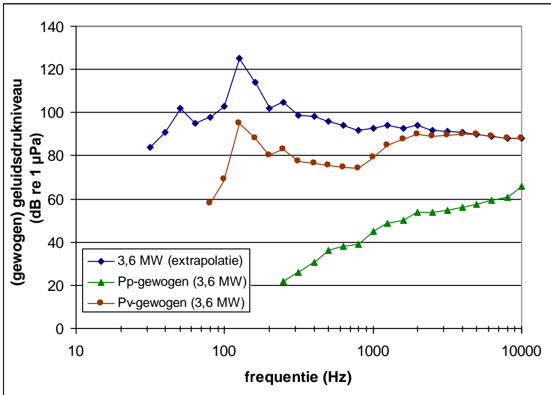
Figuur 16: op metingen in het windpark Paludans Flak gebaseerde ongewogen en audiogram gewogen geluidsspectra op 100 m van de windturbine; frequentie in tertsbanden; Pp = Bruinviss ( Phocoena phocoena ); Pv = Gewone zeehond ( Phoca vitulina )
