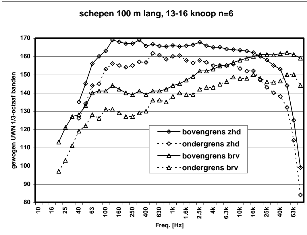
Figuur 26: spreidingsgebied van het uitgestraald geluid van 6 koopvaardij-schepen met een lengte van ca. 100 m en een vaarsnelheid tussen 13 – 16 knoop. Voor zeehond en Bruinvis gewogen bronniveau in 1/3-octaf banden en in dBw re 1 \mu\text{Pa}^2 \text{m}^2 .
