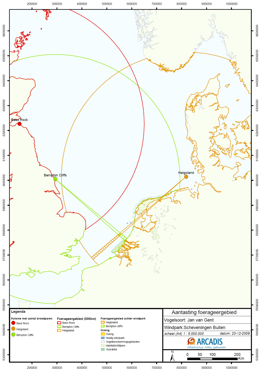
Figuur 19: Effectgebied Jan van gent vanuit (Natura 2000) broedkolonies, voor het windpark Scheveningen Buiten. Weergegeven is de maximale actieradius van Jan van genten vanuit verschillende kolonies langs de Noordzee. Aangezien de vogels die achter het windpark foerageren een verhoogd aanvaringsrisico hebben behoren deze (gearceerde) gebieden net als het windpark tot het 'effectgebied'.
