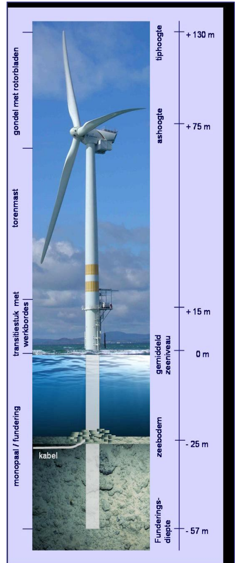
Figuur 3: opbouw van de windturbine (3.6 MW)
