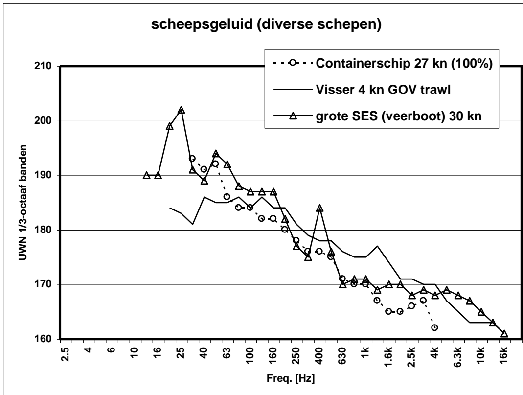
Figuur 25: de gemiddelde bronniveaus ( L_{eq} ) van diverse schepen, gemeten in 1/3-octAAF bandbreedte en in dB re 1 \mu\text{Pa}^2 \text{m}^2 .
