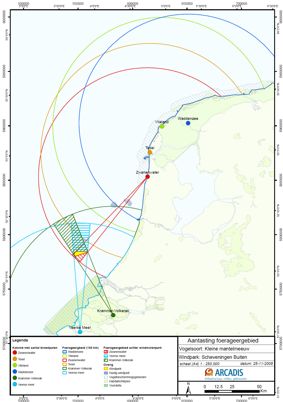
Figuur 18: Effectgebied Kleine mantelmeeuw vanuit Nederlandse (Natura 2000) broedkolonies, voor het windpark Scheveningen Buiten. Weergegeven is de gemiddelde maximale foerageer afstand van Kleine mantelmeeuwen vanuit verschillende kolonies in de Nederlandse kustzone. Aangezien de vogels die achter het windpark foerageren een verhoogd aanvaringsrisico hebben behoren deze (gearceerde) gebieden net als het windpark tot het 'effectgebied'.
