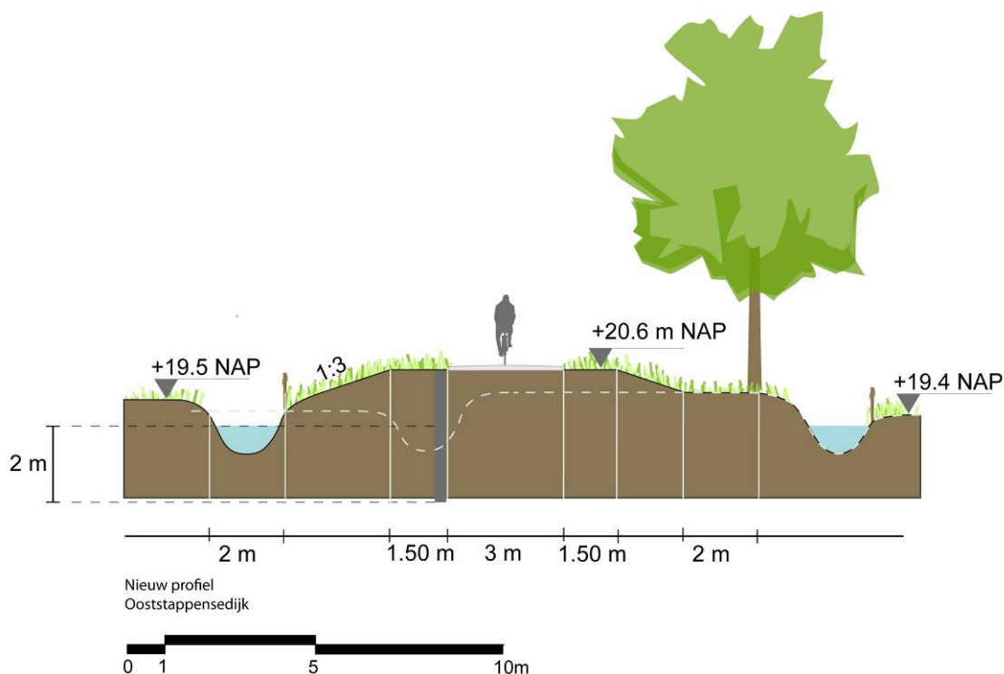
Figuur 3.4. Dwarsprofiel kade Oostappensedijk (lokaal opgehoogd wegtracé, behoud van monumentale beplanting)
