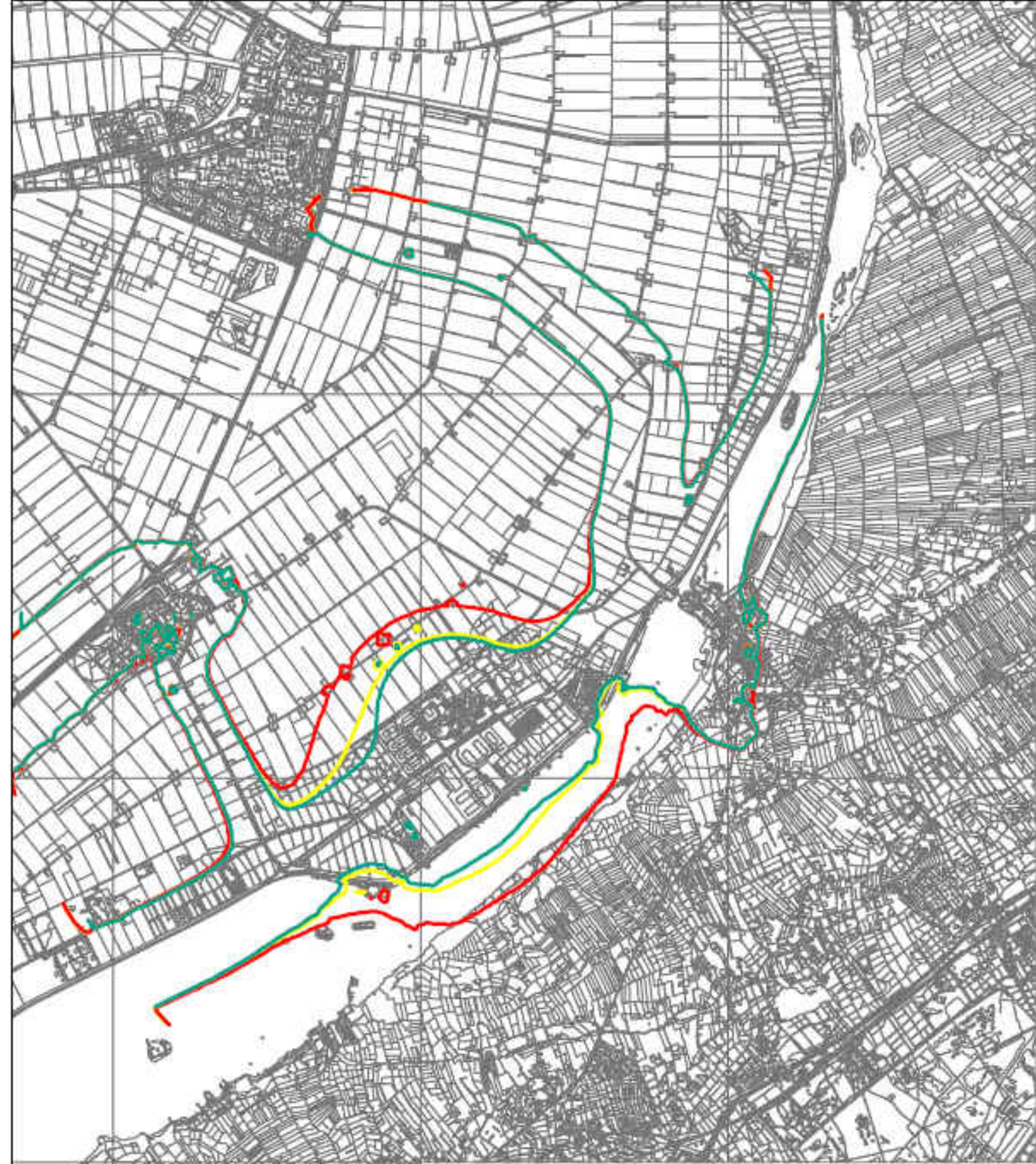
36 dB contour op 4 meter hoogte voor de verschillende situaties Maximale variant
